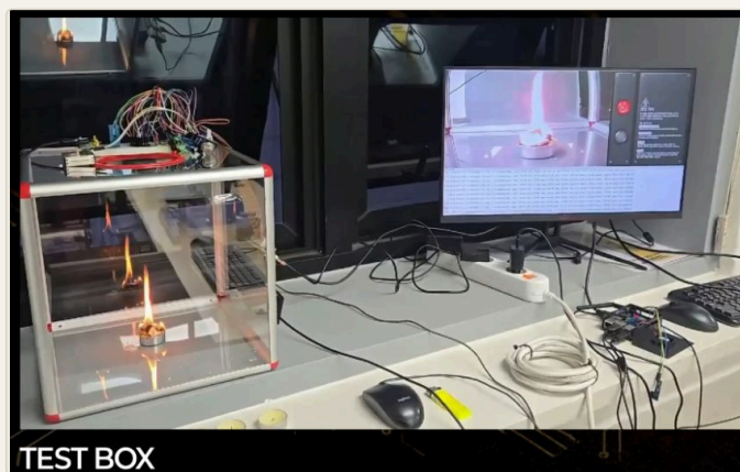
현장 사진 / PRISM — 테스트 박스 화재 시험과 같은 순간의 관제 대시보드
