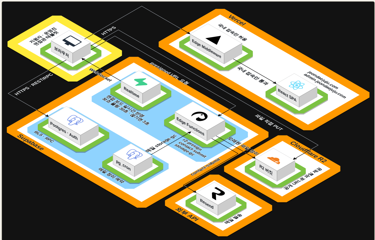
아키텍처 / 전대주주 플랫폼 시스템 아키텍처 — Vercel · Supabase · Cloudflare R2
