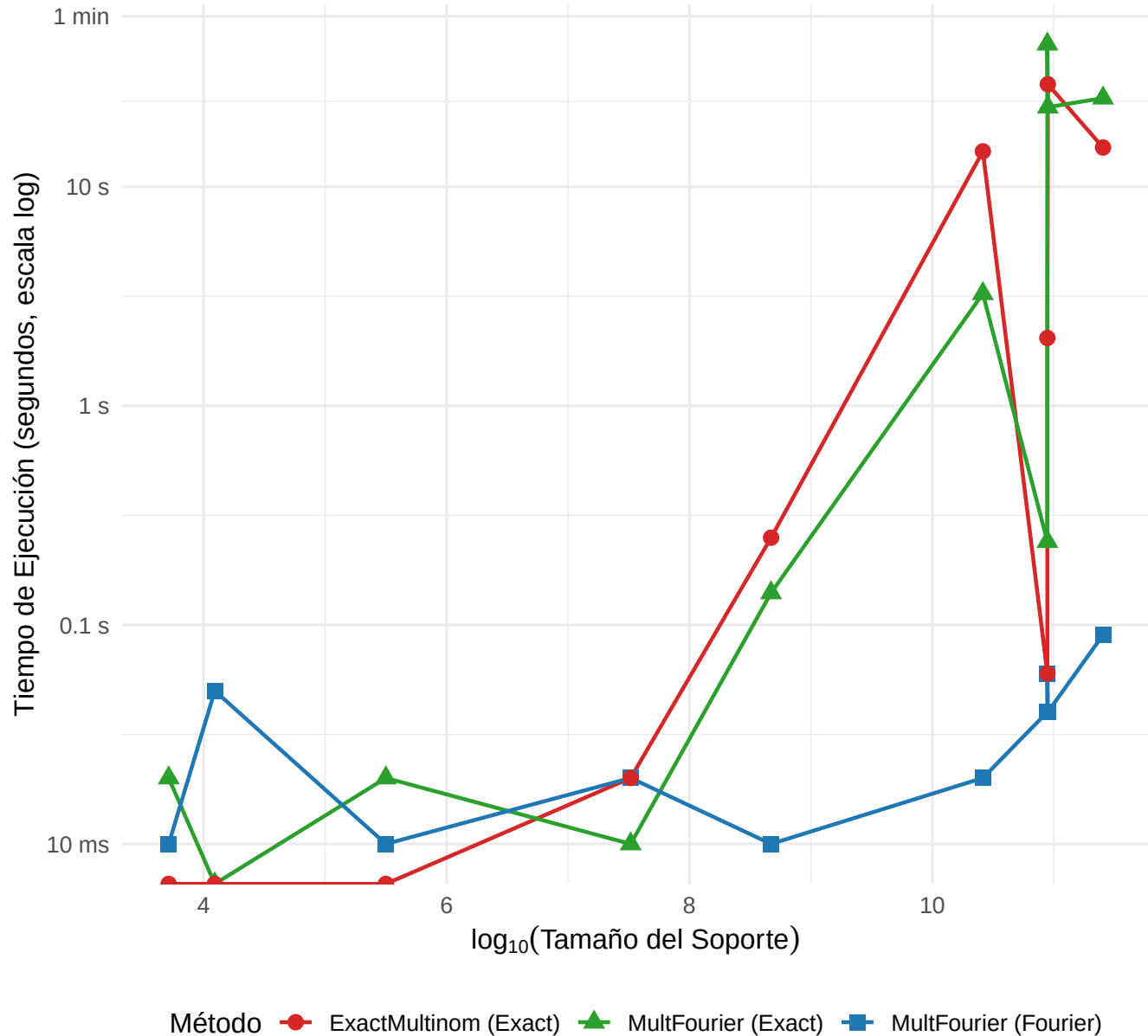
Tiempo de Cómputo vs. Tamaño del Soporte Multinomial Comparación entre MultFourier (Fourier y Exact) y ExactMultinom
