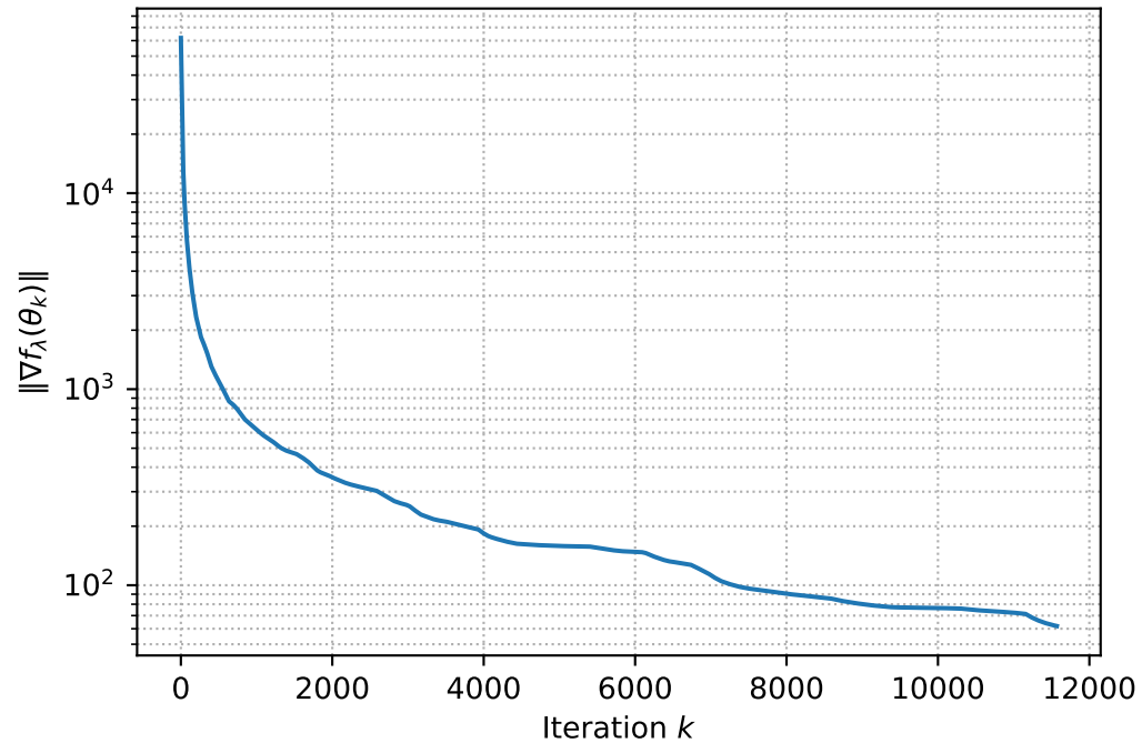
Gradient norm
