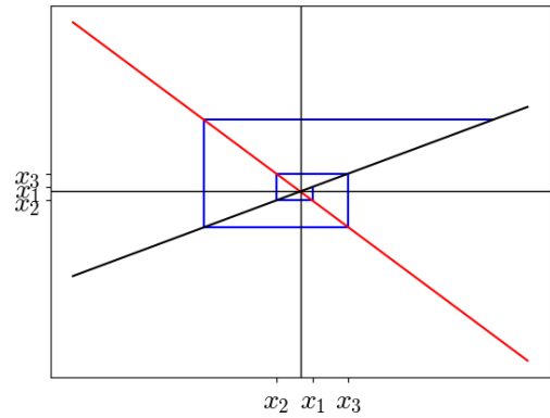
(d) Cobweb diagram for the function f(x) = ax when a = -2
