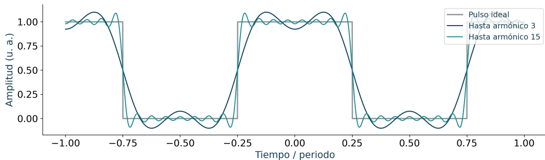
Figura 2: Pulso sintético de ciclo de trabajo 1/2. Aumentar armónicos estrecha la región de Gibbs, pero no elimina su sobreimpulso relativo.
