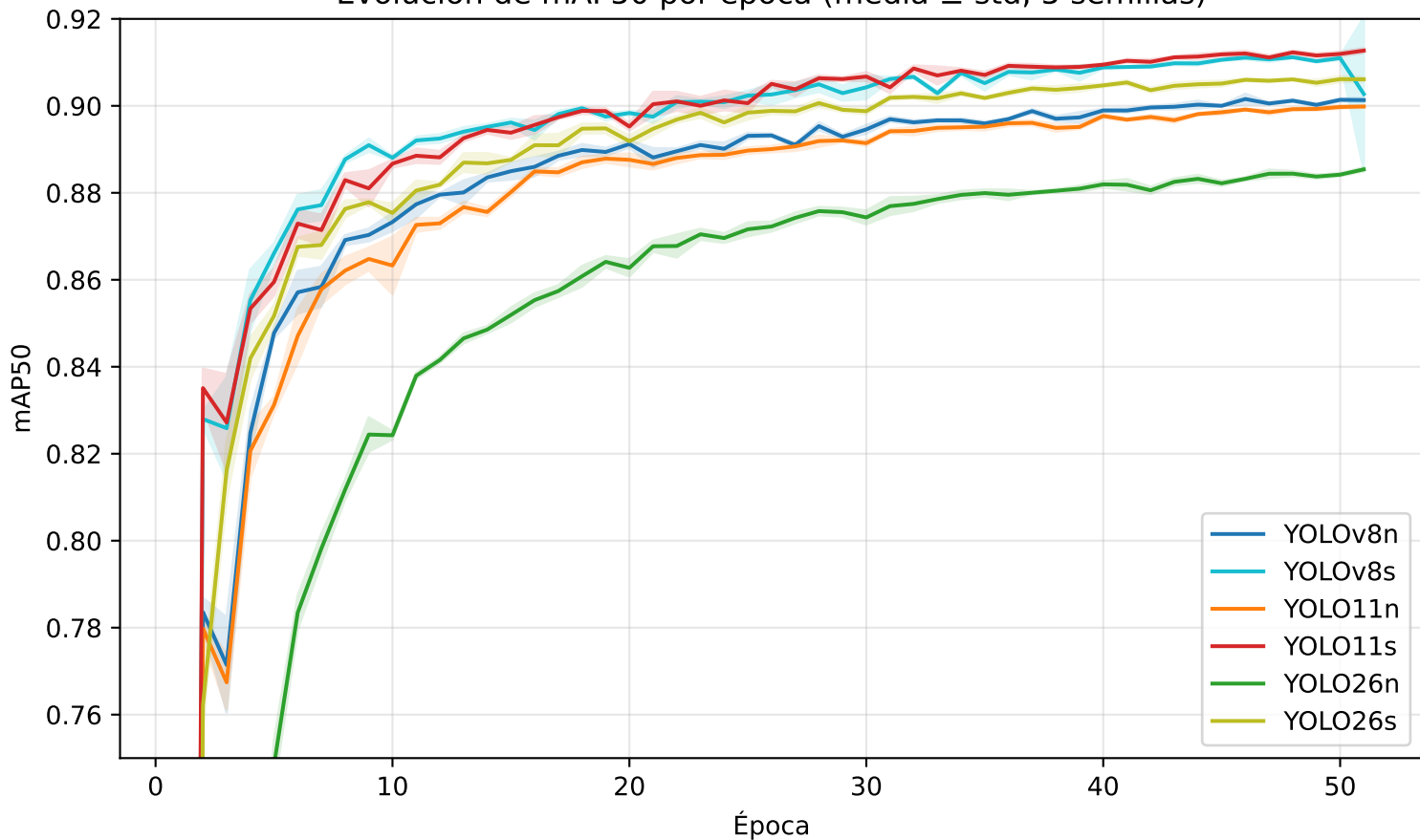
Evolución de mAP50 por época (media \pm std, 5 semillas)
