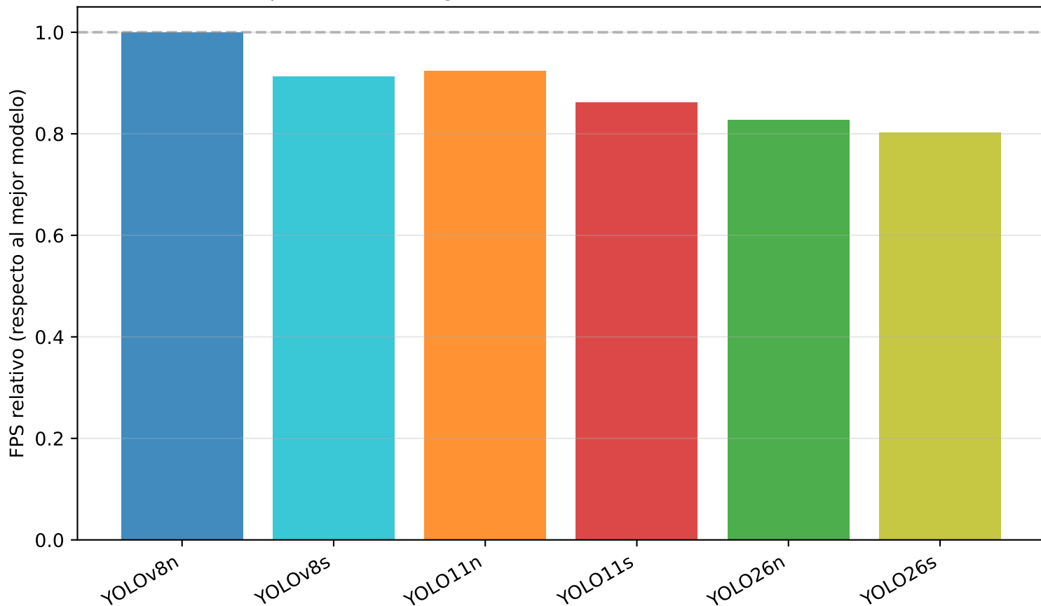
FPS relativo por modelo (imgsz=640, batch=1, NVIDIA GeForce RTX 3060 Ti)
