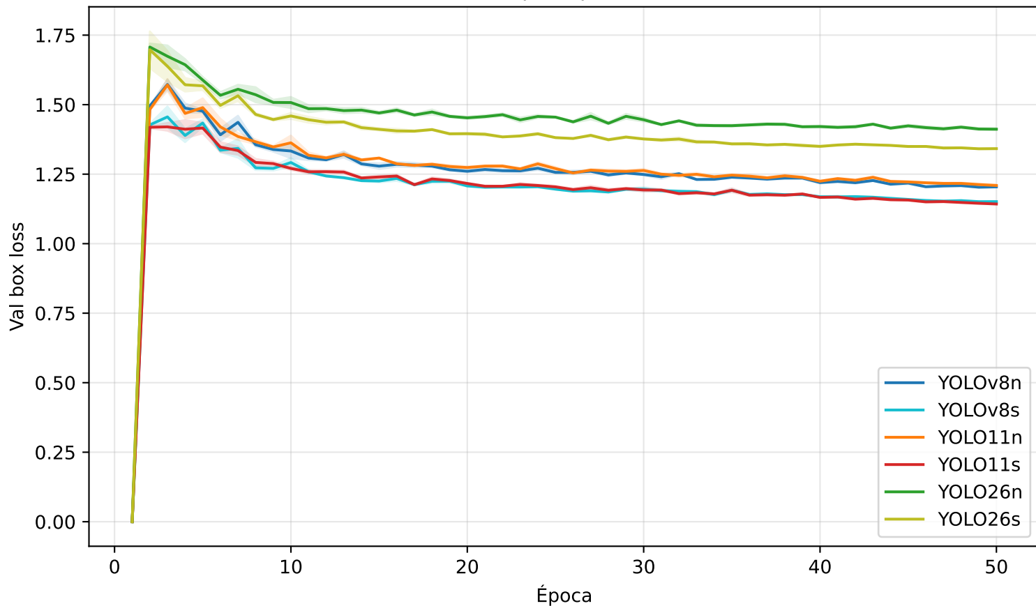
Evolución de la val box loss por época (media \pm std, 5 semillas)
