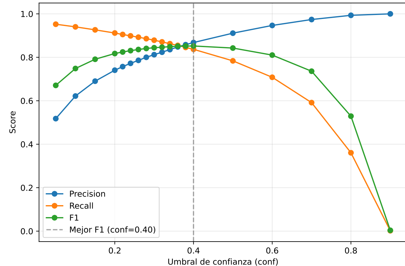
Precision / Recall / F1 vs umbral de confianza
