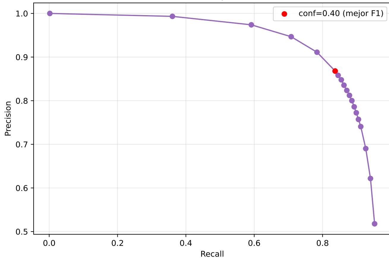
Curva Precision-Recall (por umbral de conf)
