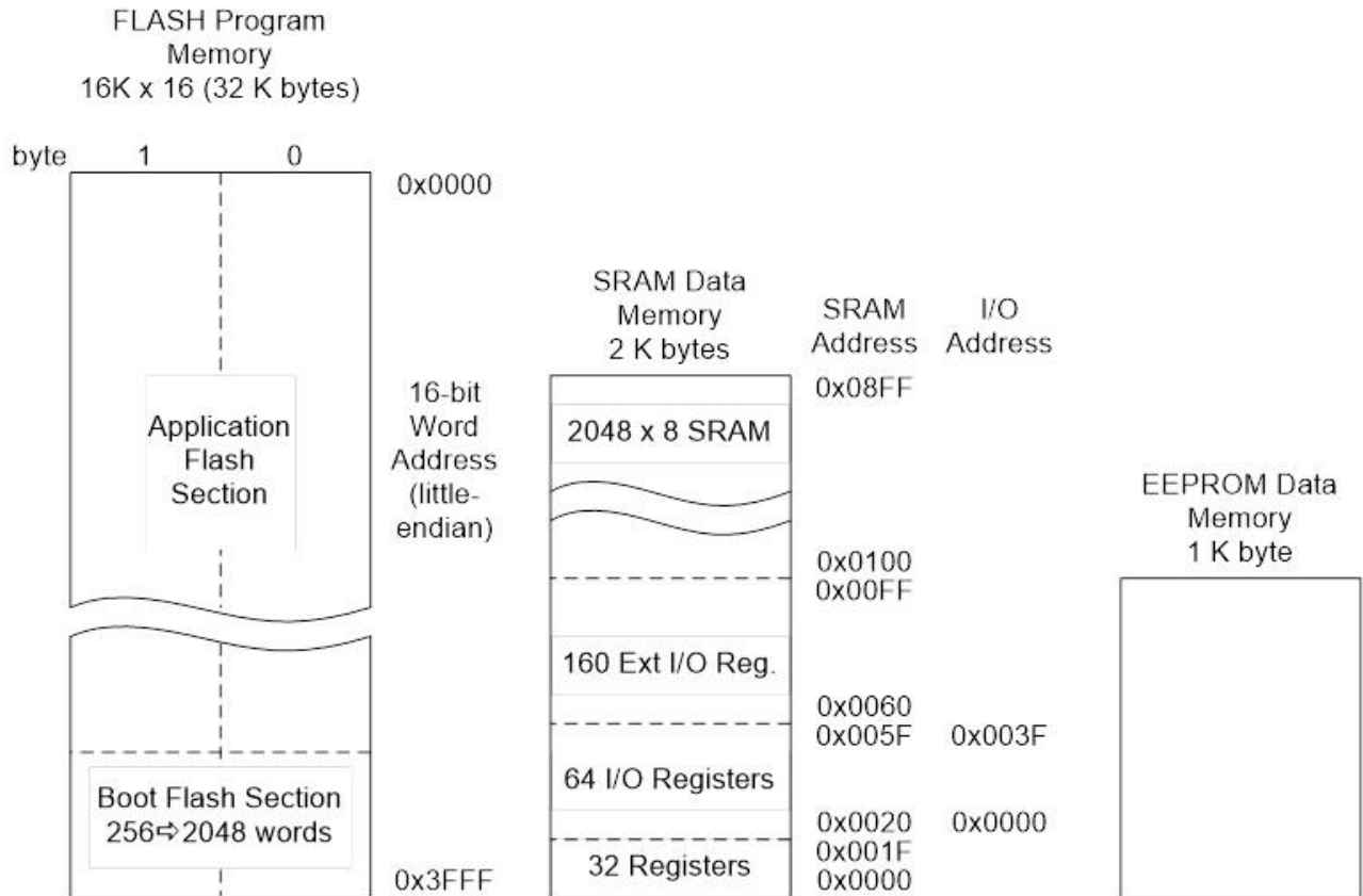
Mapa de memoria de un ATmega 328,
