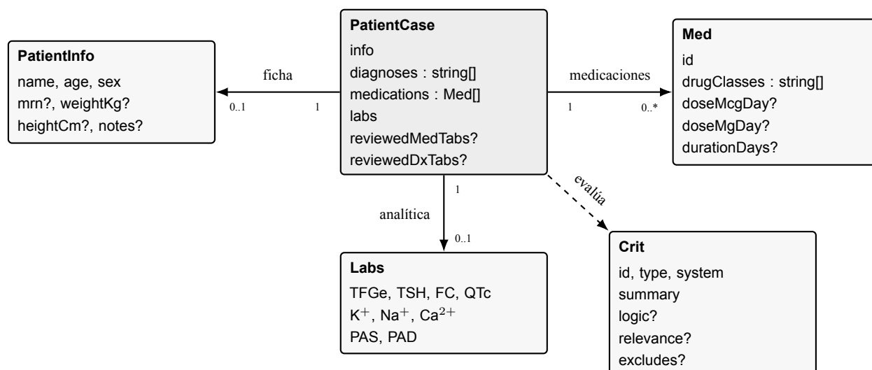
Figura 8.1: Modelo de dominio simplificado. Crit no se persiste con el caso: el motor lo produce al evaluar.
