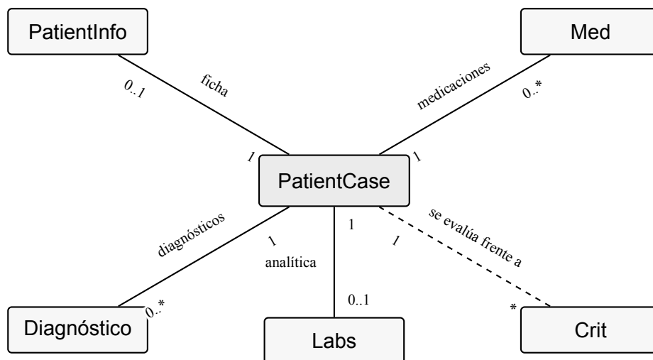
Figura 7.2: Entidades del dominio, con el nombre de cada relación sobre la línea y las multiplicidades en los extremos. Crit pertenece al catálogo; el resto constituye el caso de sesión.
