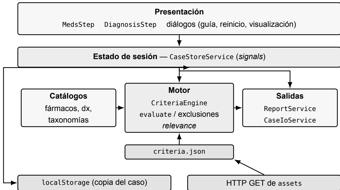
Figura 5.1: Arquitectura de cajas: la UI actualiza el estado de sesión; el motor evalúa el caso con catálogos y criteria.json ; las salidas leen una instantánea. El estado vive en memoria; localStorage guarda una copia en el navegador, no en una base de datos. HttpClient obtiene los activos mediante HTTP GET.
