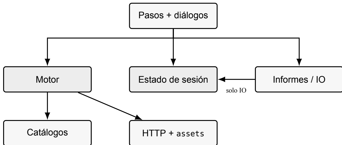
Figura 5.2: Dependencias lógicas: los pasos orquestan; el motor no depende de la UI; solo el servicio de intercambio JSON accede directamente al estado de sesión. Ese estado no es una base de datos.
