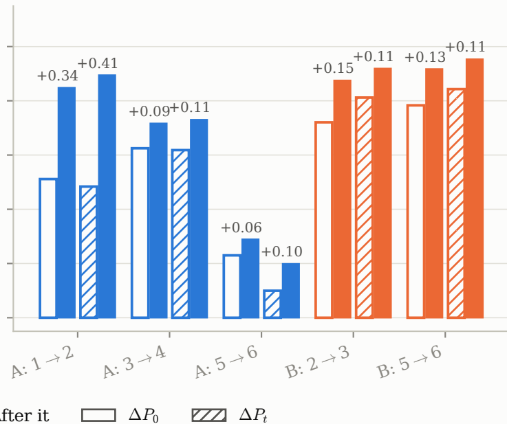
Sycophancy
