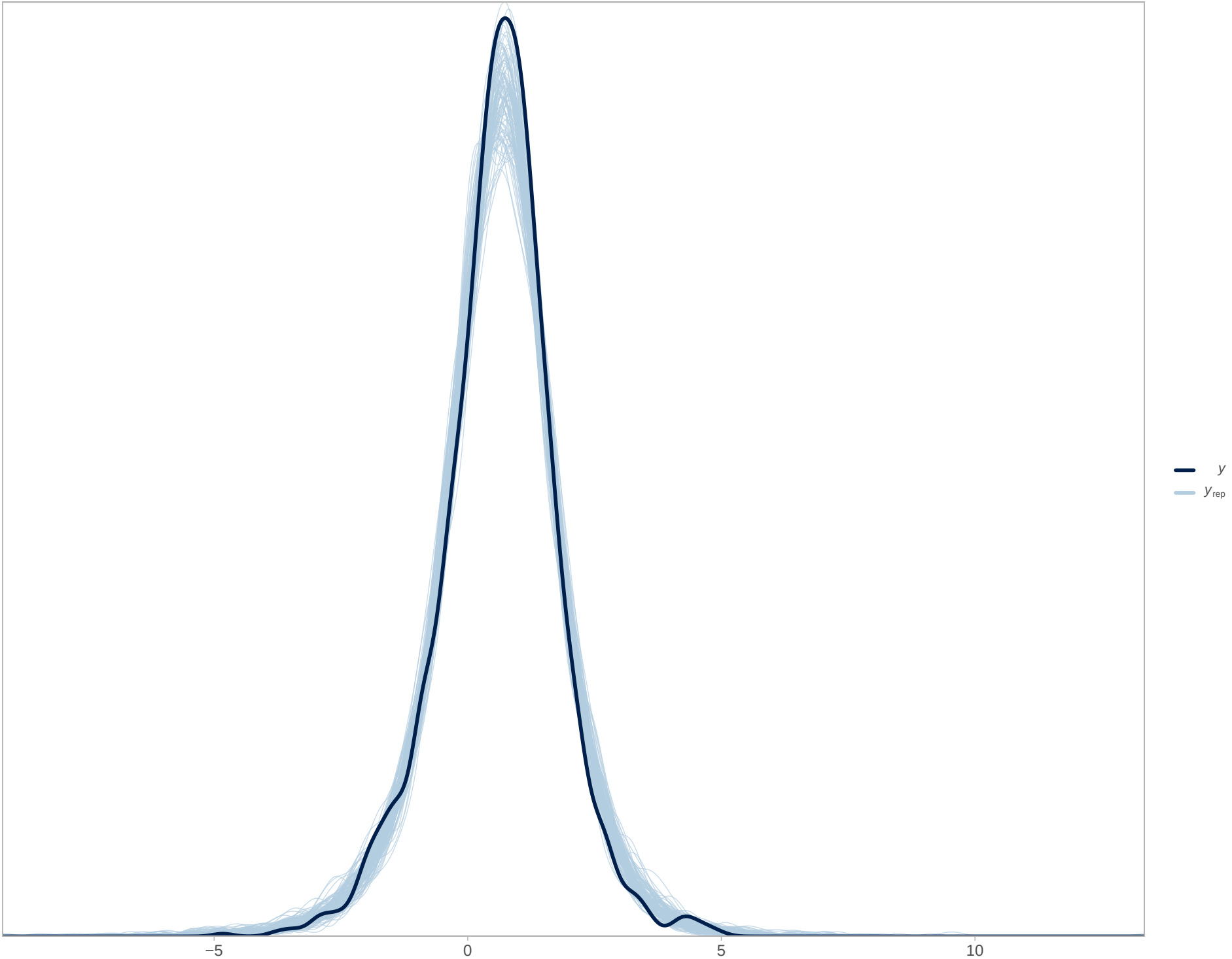
Y rep: posterior predictive check
