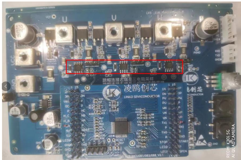
图 2.8 demo 硬件图
