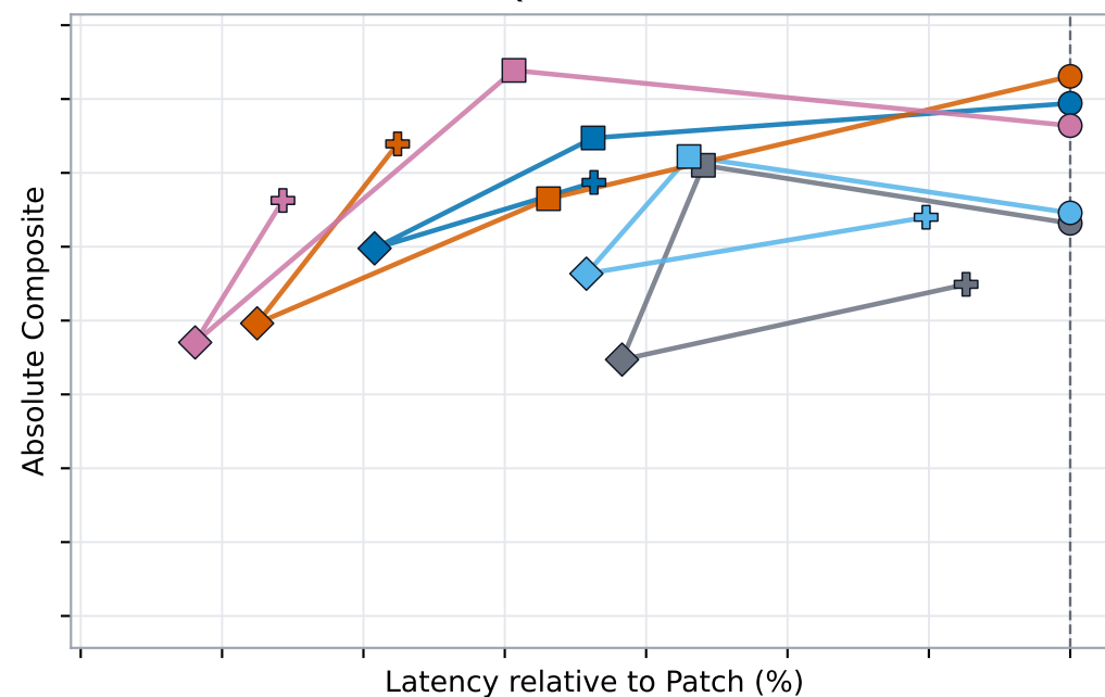
Qwen 0.8B
