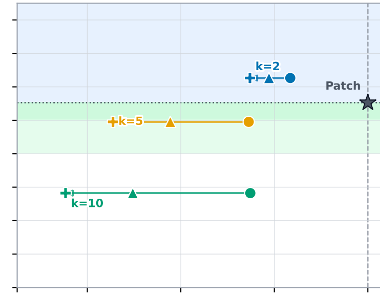
Llama 1B
