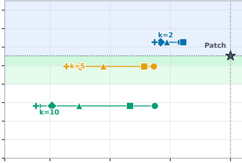
Llama 1B
