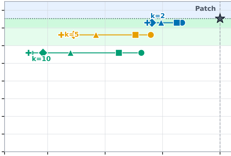
Llama 3B
