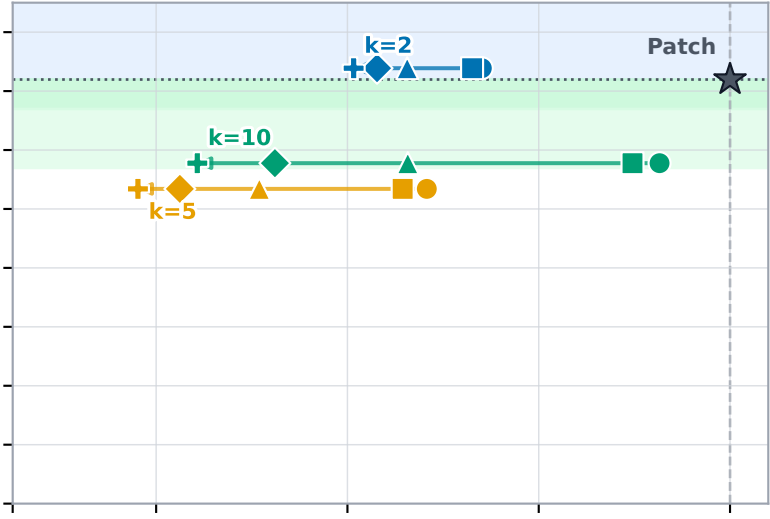
Qwen 0.8B
