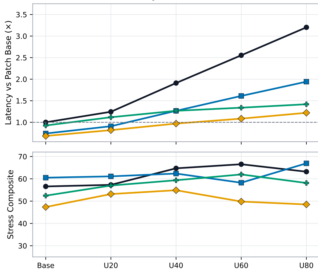
Qwen 0.8B
