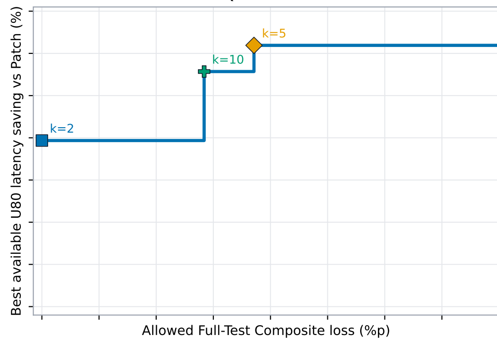
Qwen 0.8B
