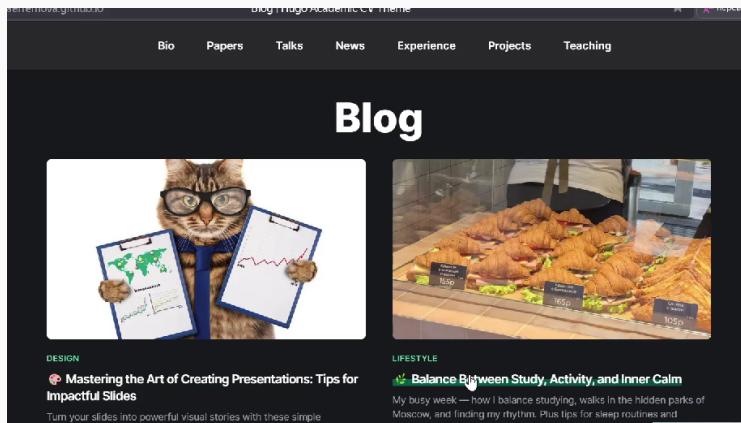
Рис. 4: Проверка постов
