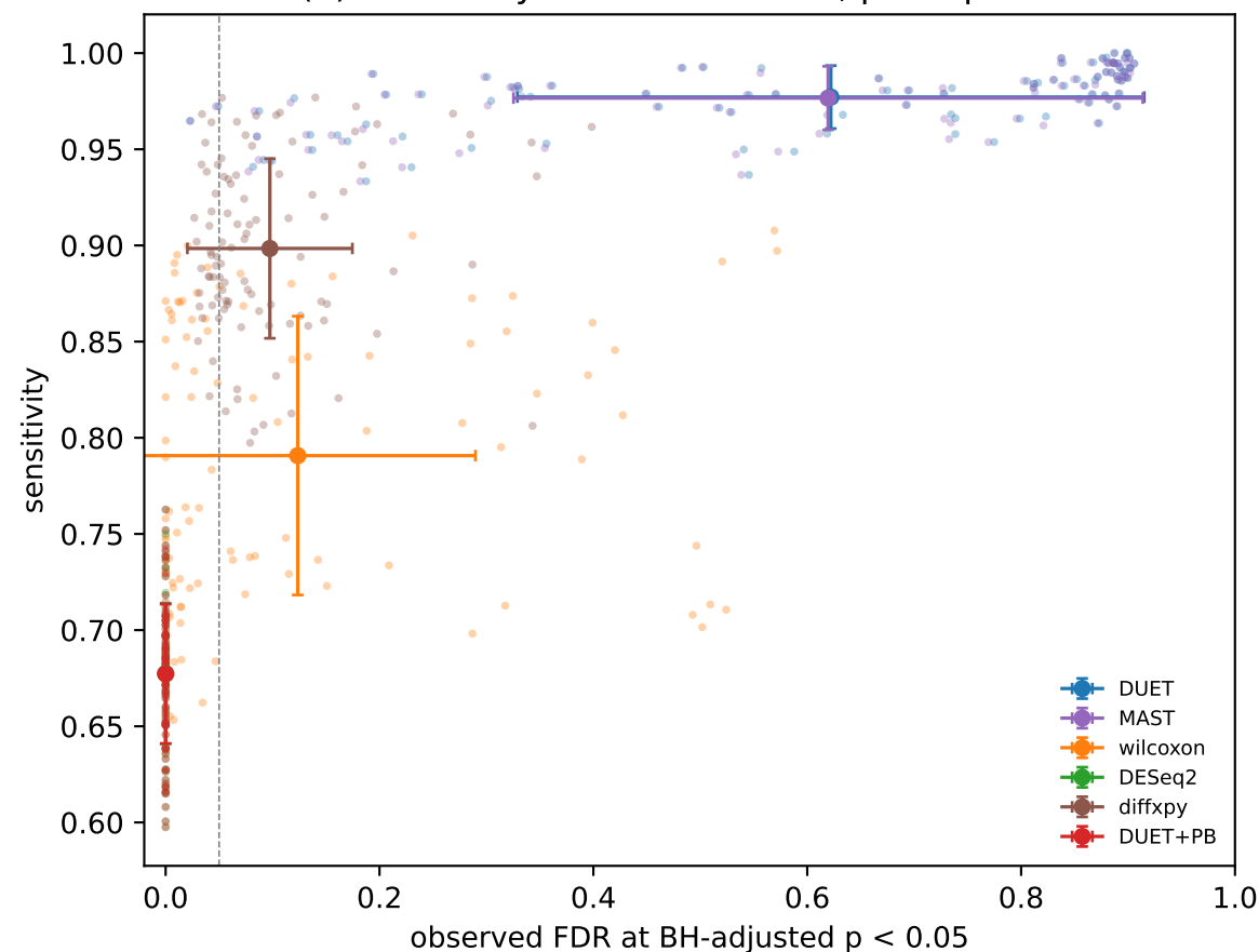
(d) donor-swap null, one point per unique partition
