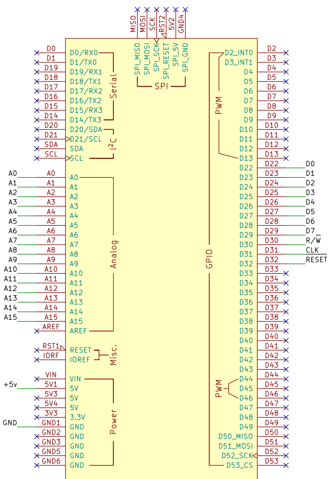
A1 Arduino_Mega2560_R3_Shield
