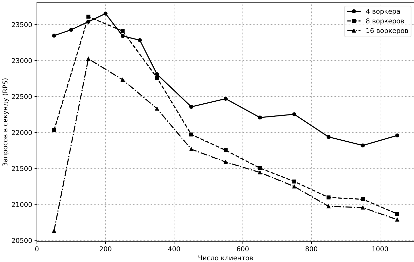
Зависимость RPS от числа клиентов
