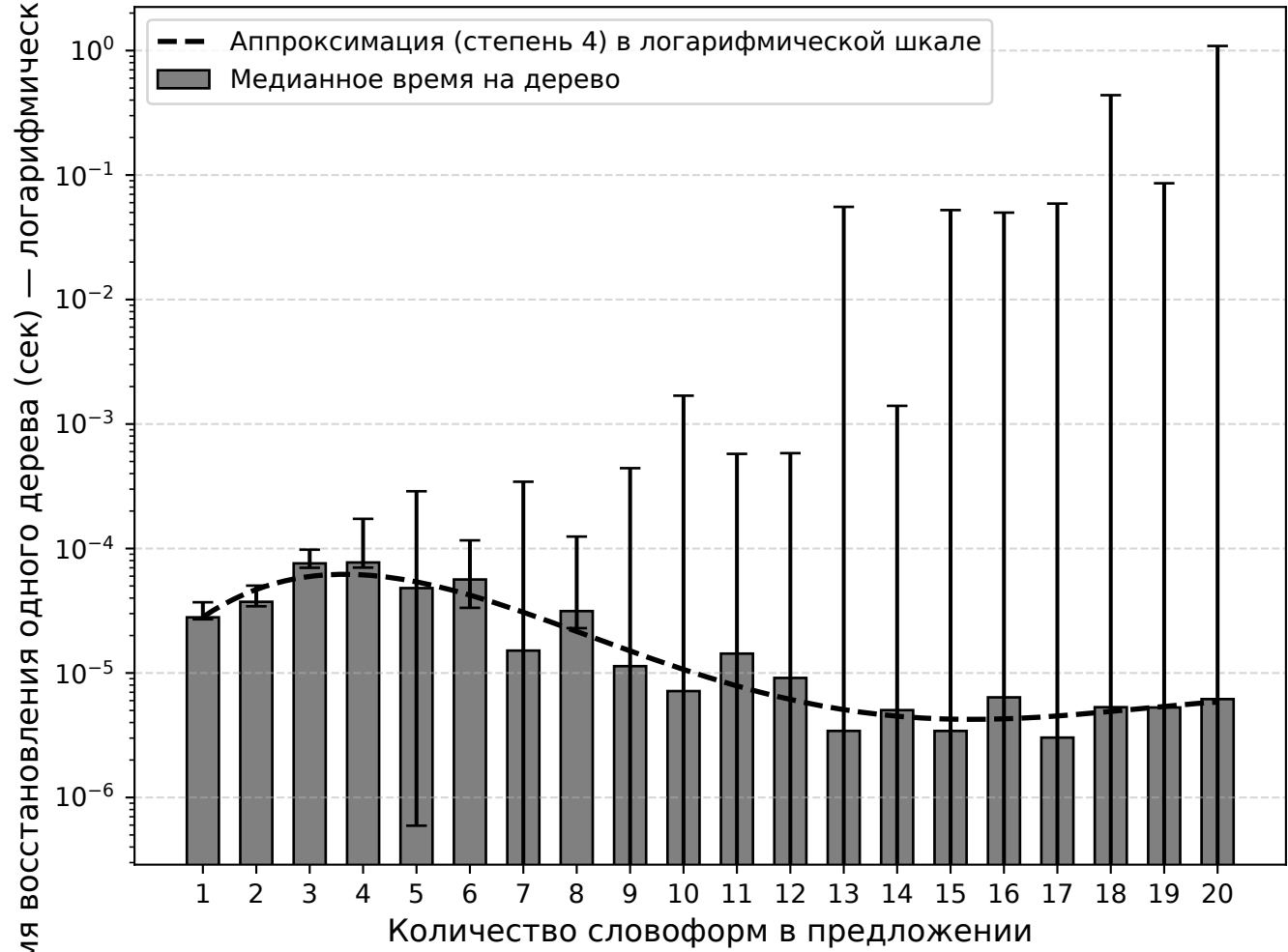
Восстановление деревьев разбора (на одно дерево, логарифмическая шкала)
