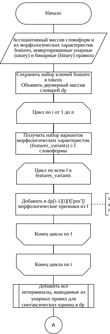
Рисунок 2.3 — Схема алгоритма построения таблицы составляющих
