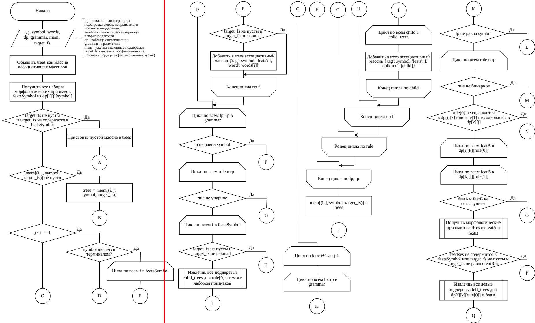
Рисунок 2.4 — Схема алгоритма восстановления дерева составляющих
