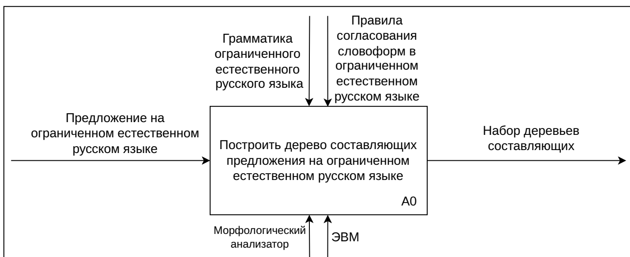
Рисунок 1.7 — IDEF0-диаграмма уровня A0
