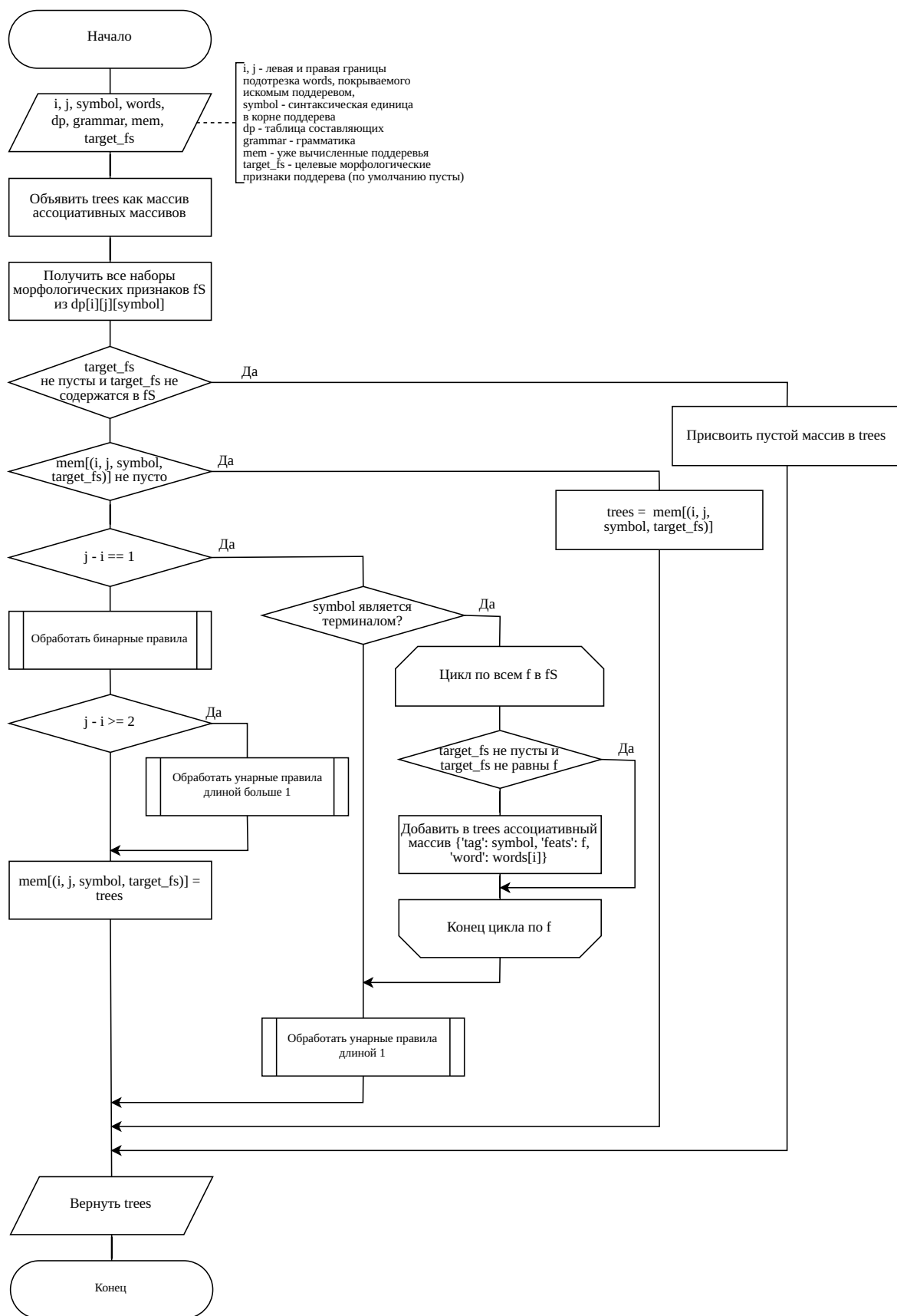
Рисунок 2.5 — Схема алгоритма восстановления дерева составляющих
