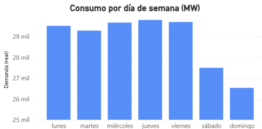
Figura 15. Consumo medio según día de la semana.
