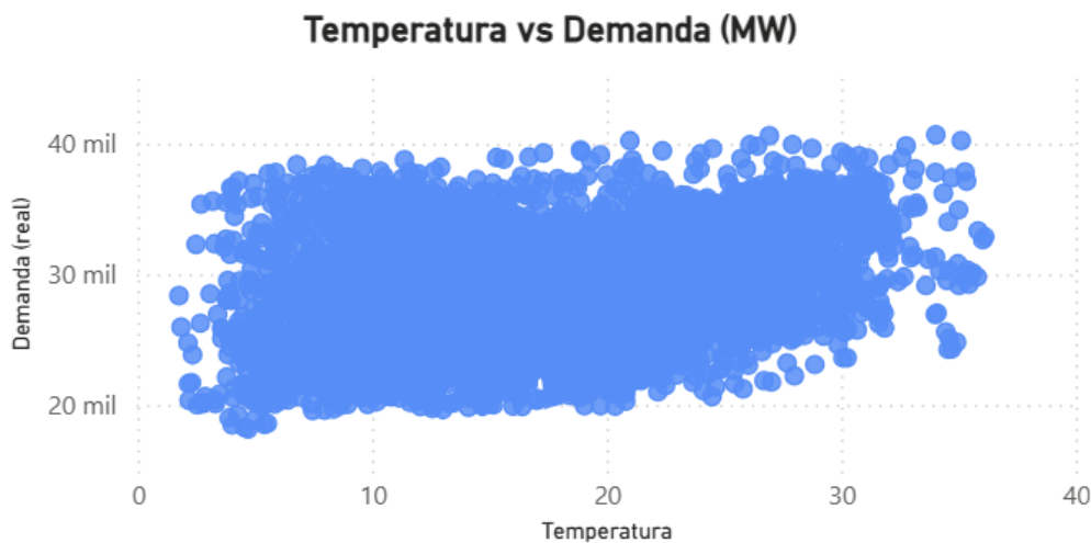
Figura 16. Relación entre temperatura y demanda eléctrica.
