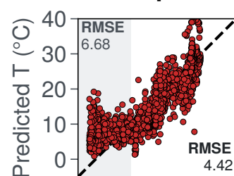
1:1 plot
