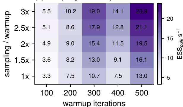
(d) sampling efficiency
