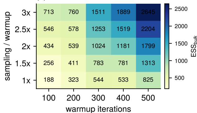
(d) sampling efficiency
