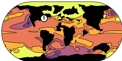
iPETM \Delta T (6x minus 3x \text{CO}_2 )
