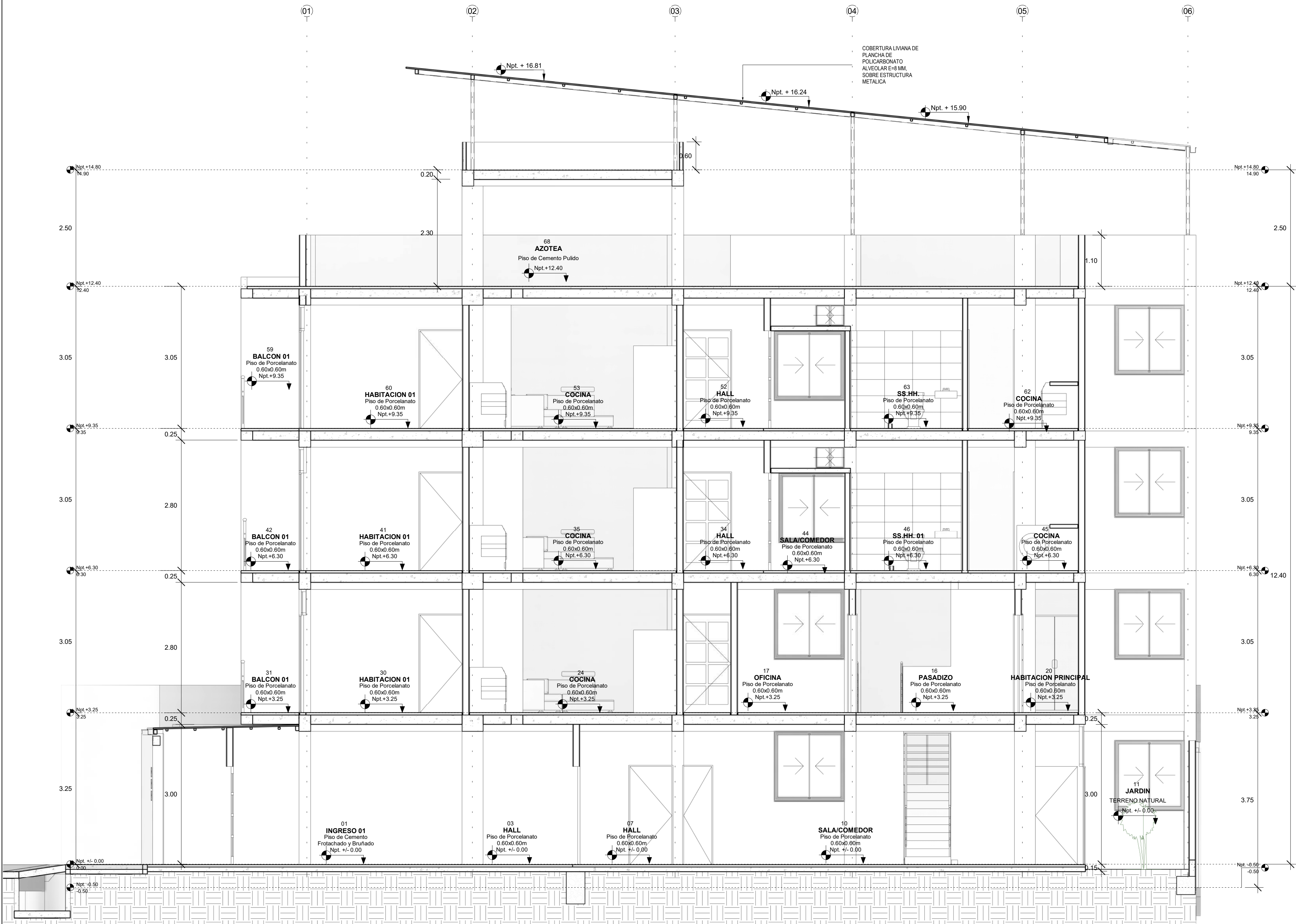
B CORTE LONGITUDINAL B-B A-05 1:50
