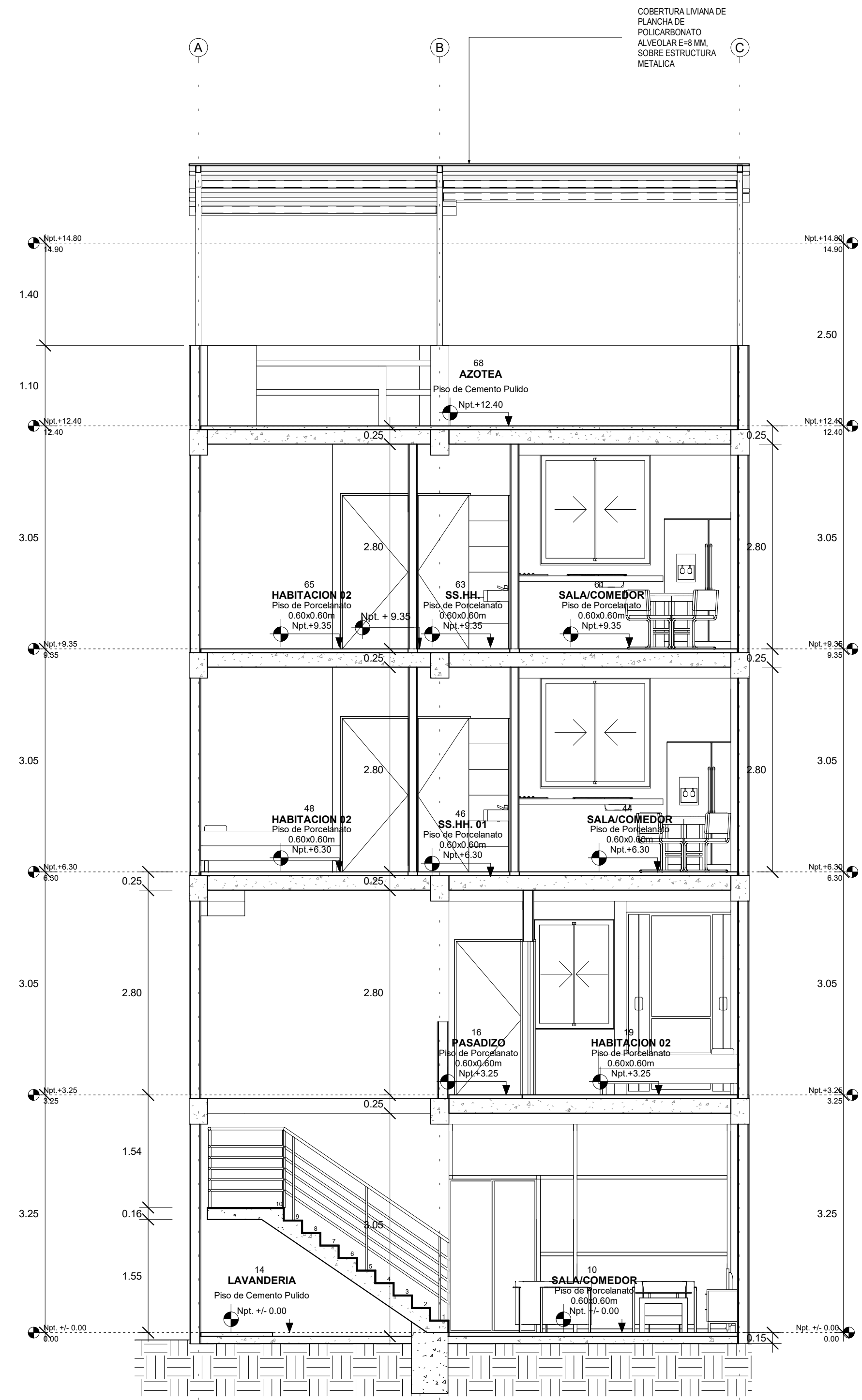
F CORTE TRANSVERSAL F-F A-06 1: 50
