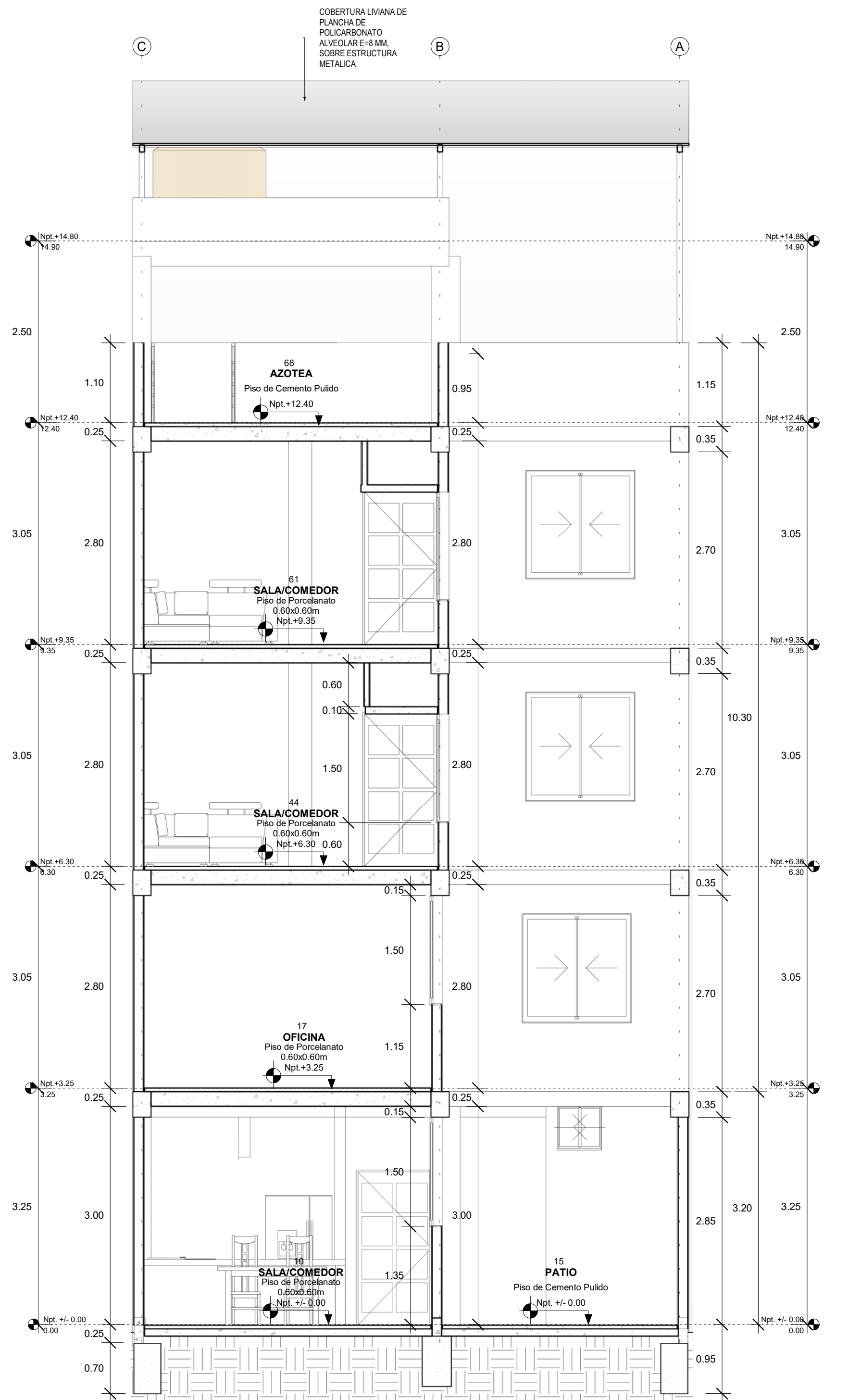
E CORTE TRANSVERSAL E-E A-05 1:50
