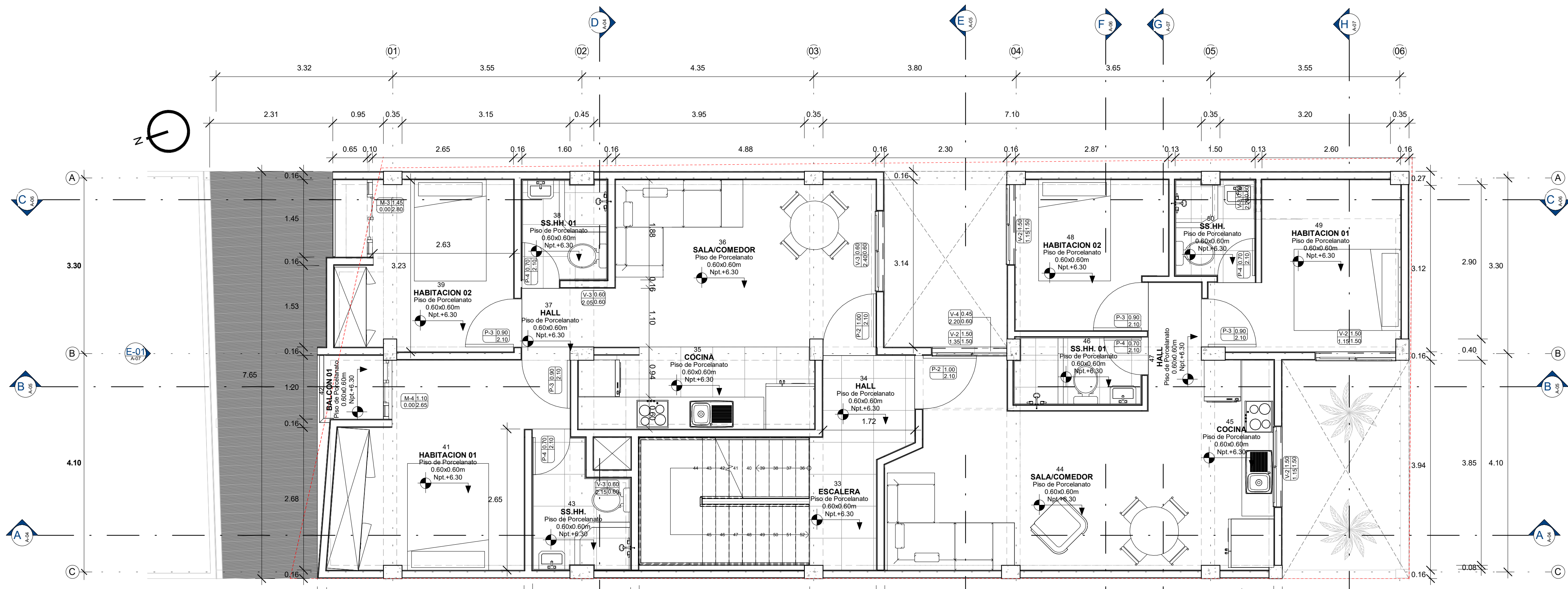
1 PLANO DE DISTRIBUCION TERCER PISO A-02 1:50
