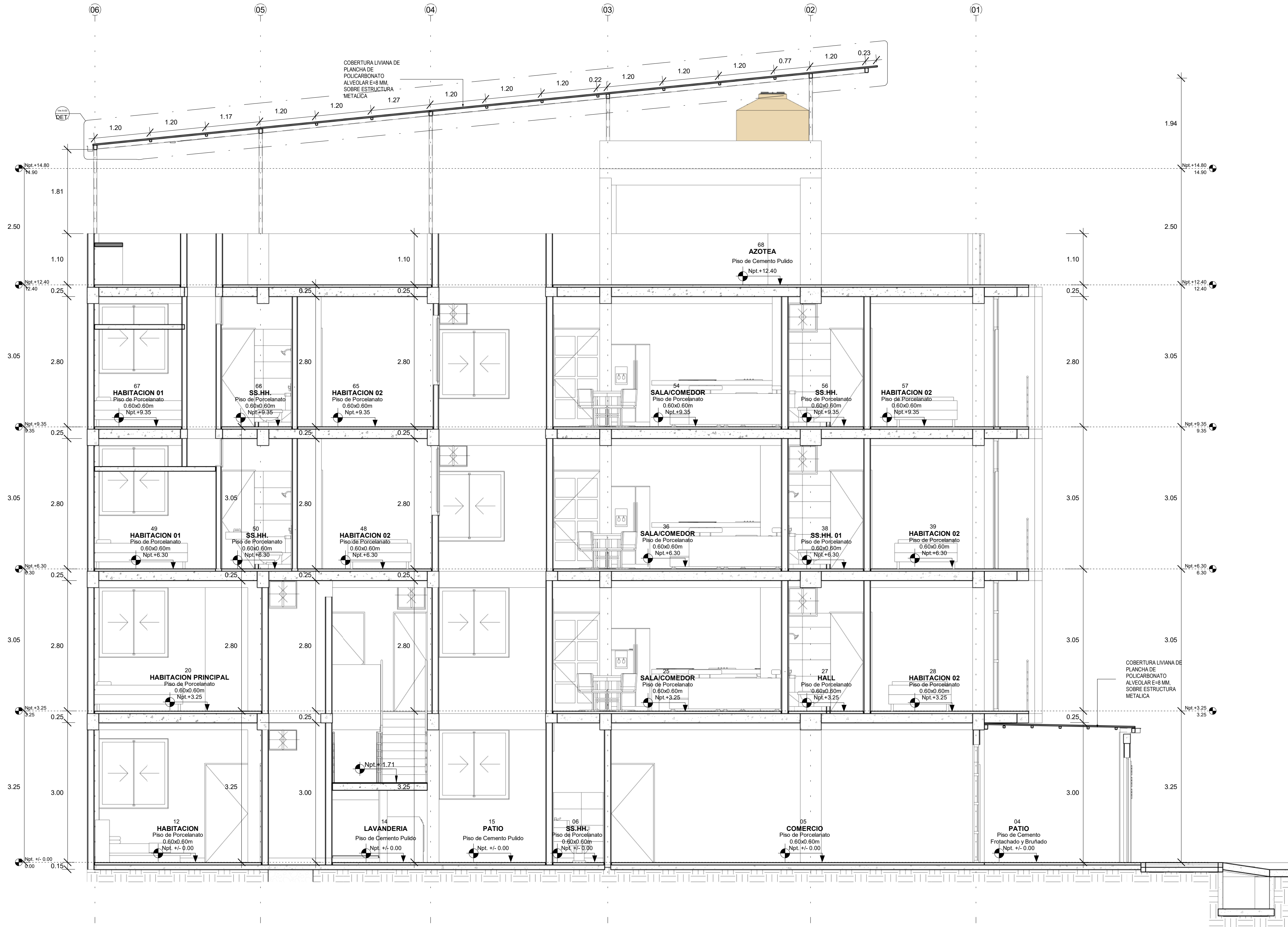
C CORTE LONGITUDINAL C-C A-06 1: 50
