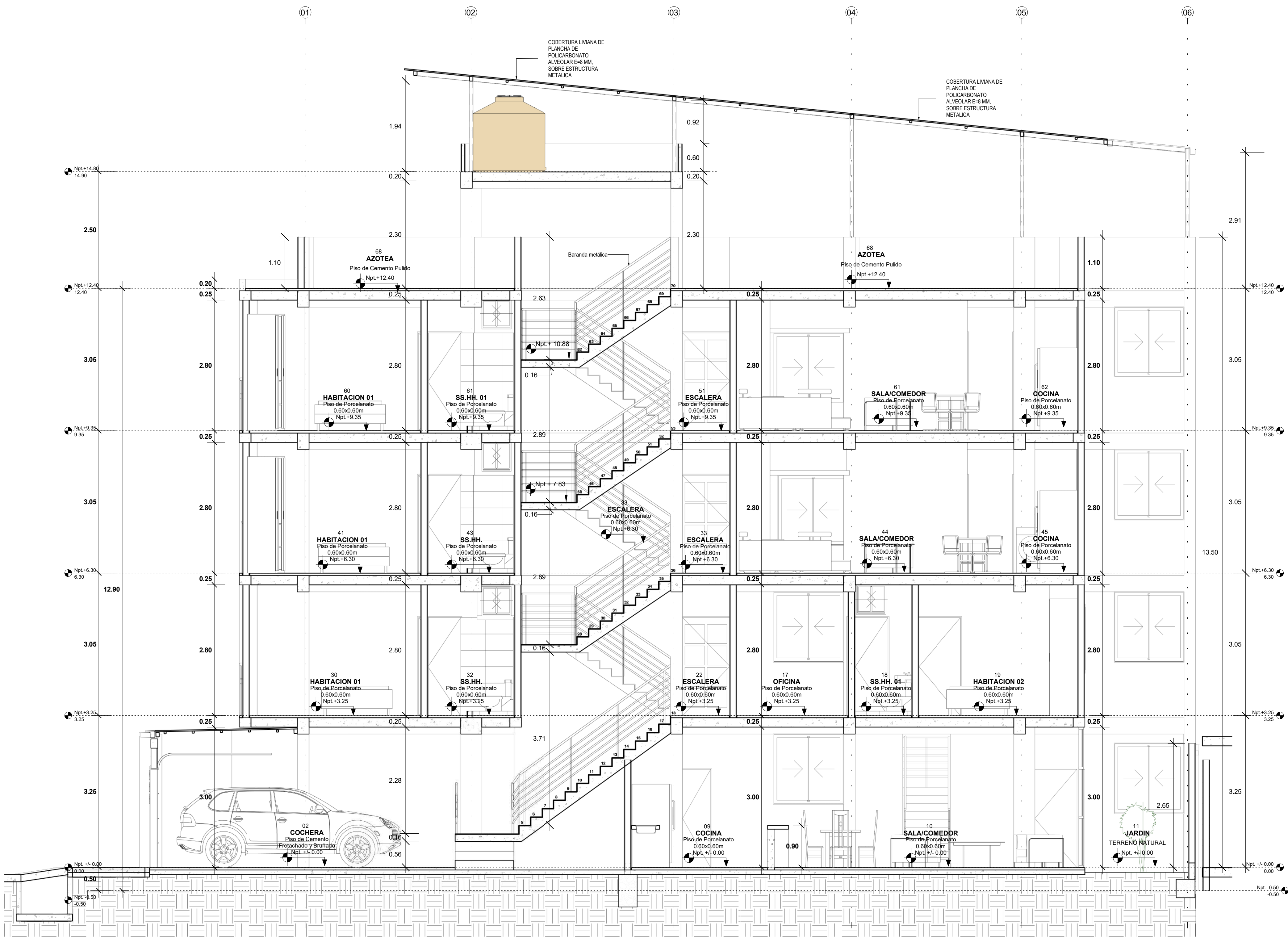
A CORTE LONGITUDINAL A-A A-04 1:50
