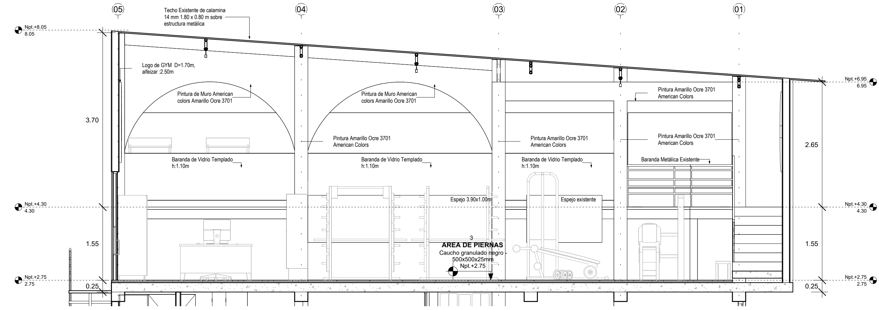
B CORTE LONGITUDINAL B-B A-02 1:50
