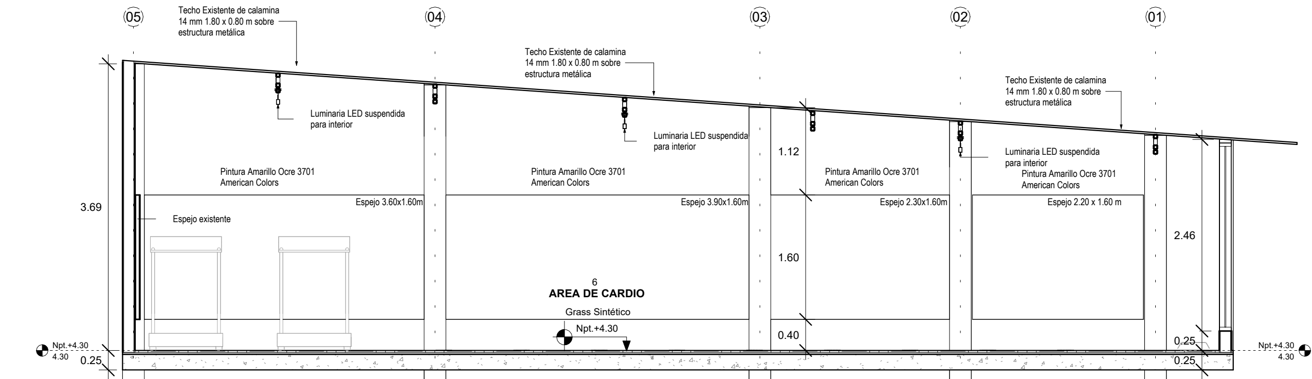
A CORTE LONGITUDINAL A-A A-02 1:50
