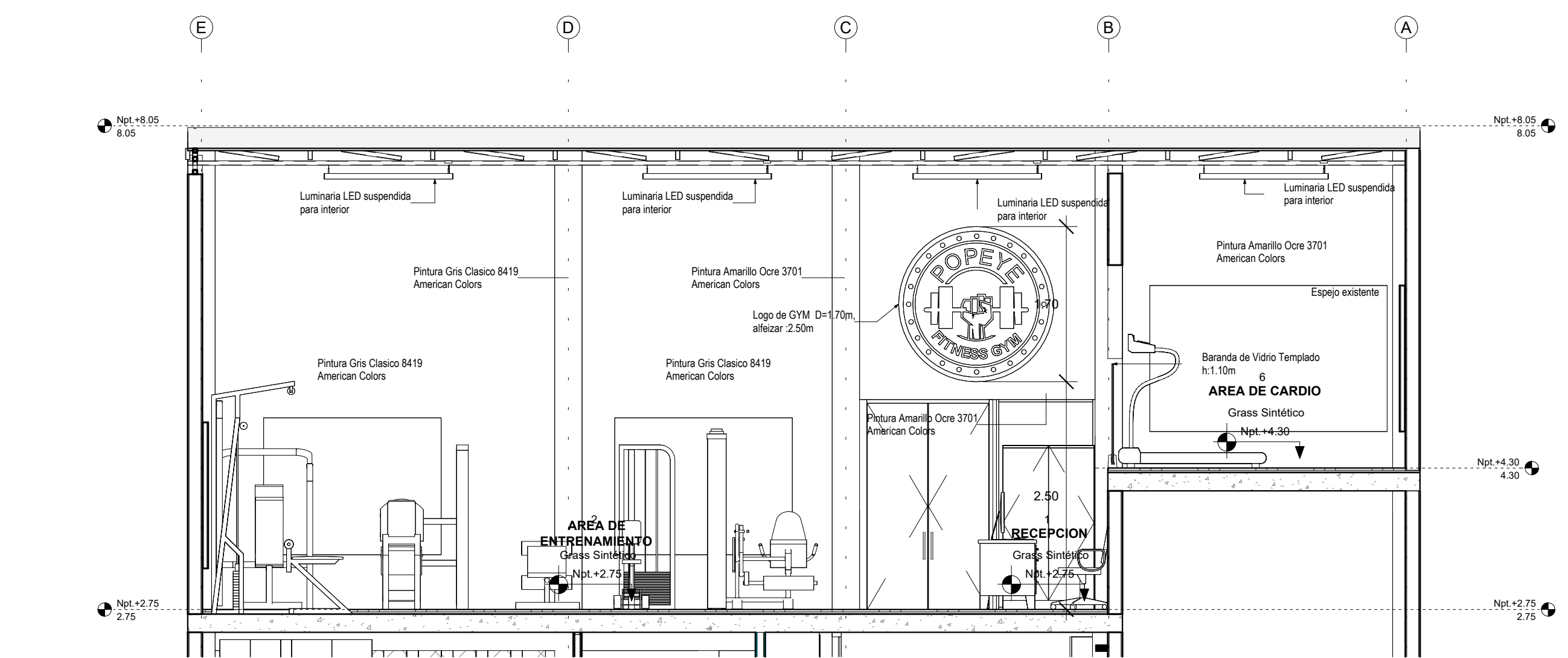
E CORTE TRANSVERSAL E-E A-02 1:50
