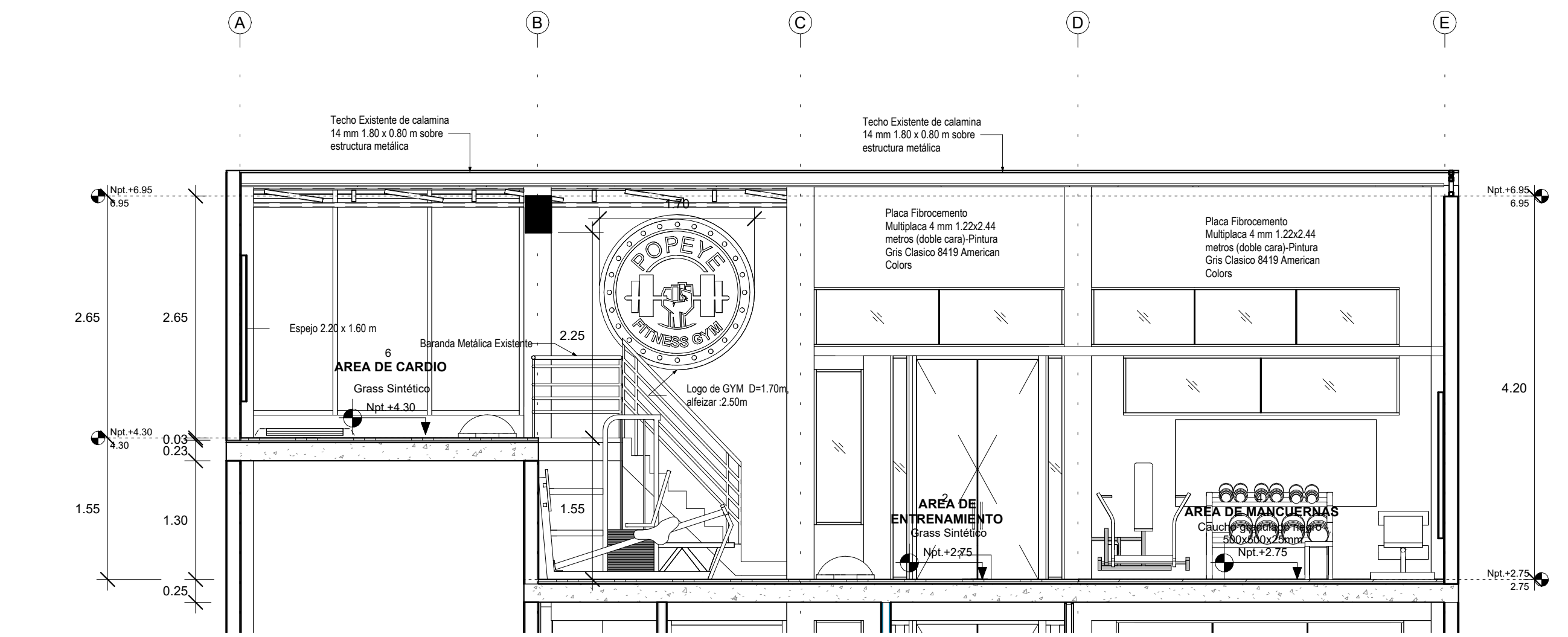
D CORTE TRANSVERSAL D-D A-02 1:50
