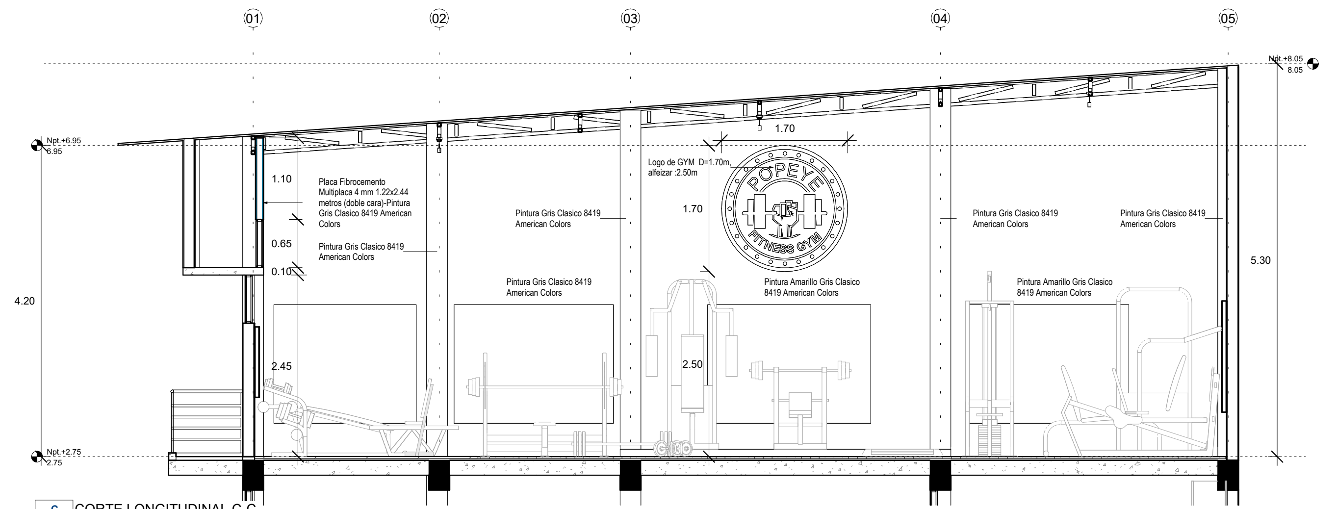
C CORTE LONGITUDINAL C-C A-02 1:50
