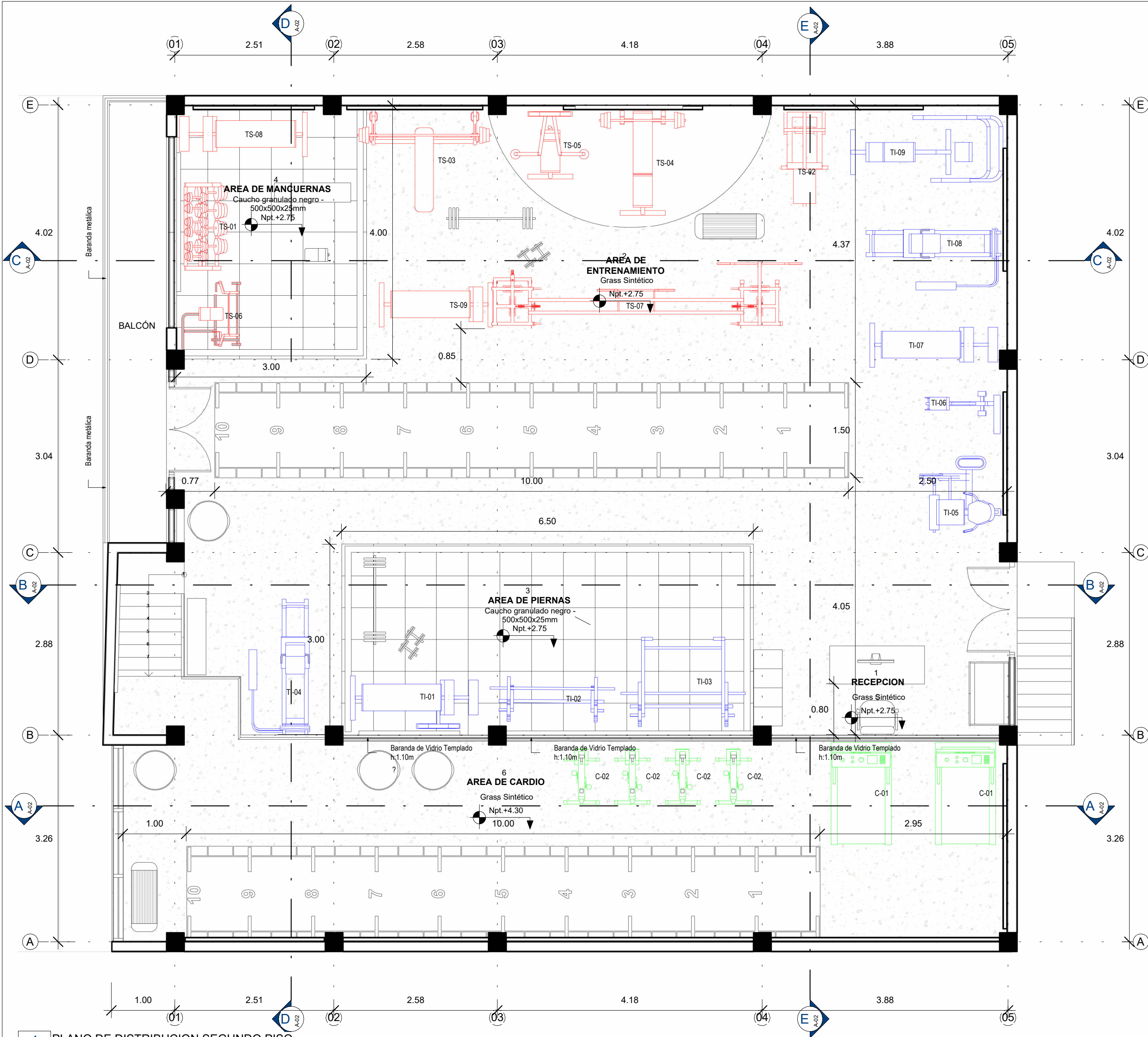
1 PLANO DE DISTRIBUCION SEGUNDO PISO A-01 1 : 50
