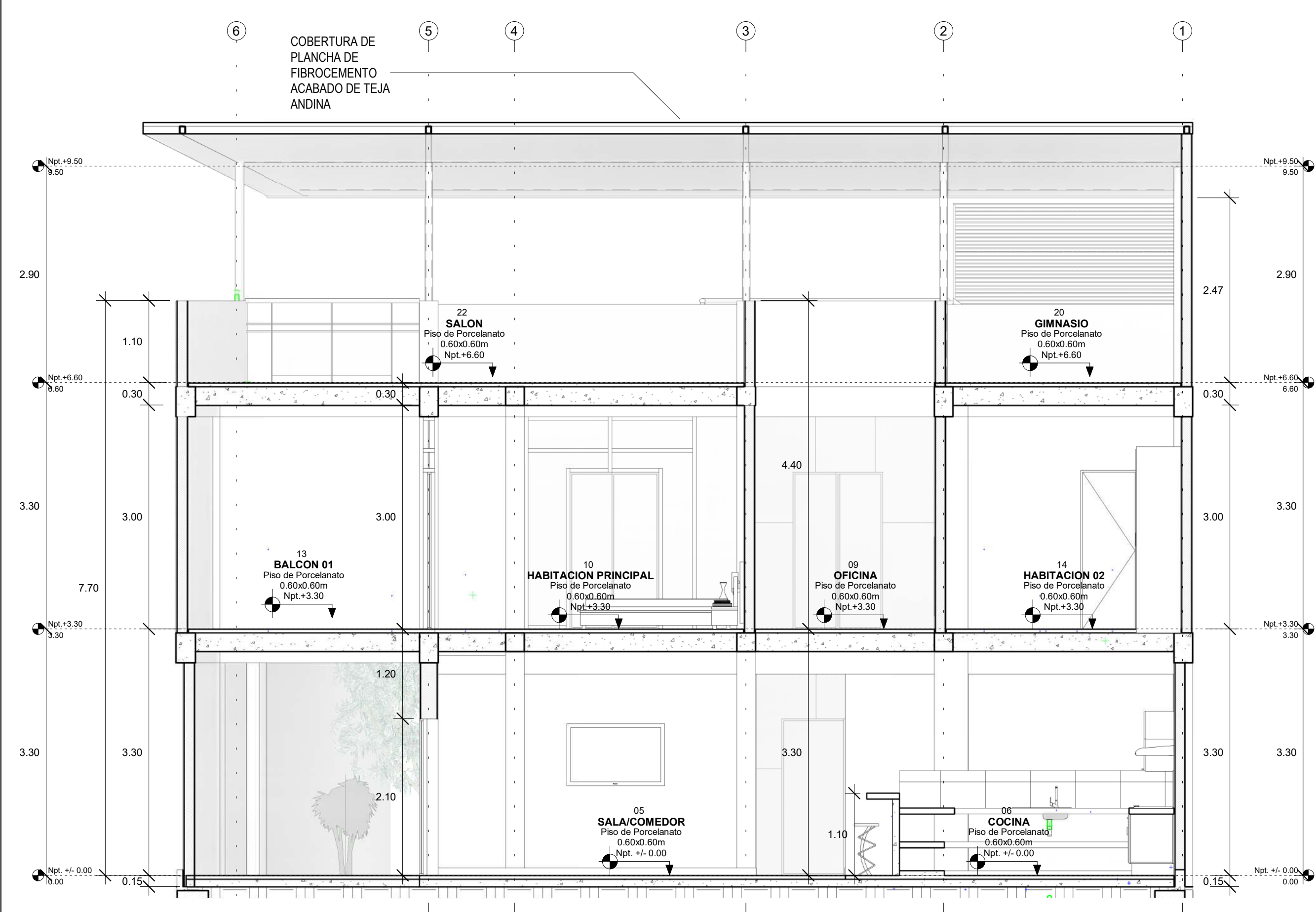
F CORTE TRANSVERSAL F-F A-06 1:50
