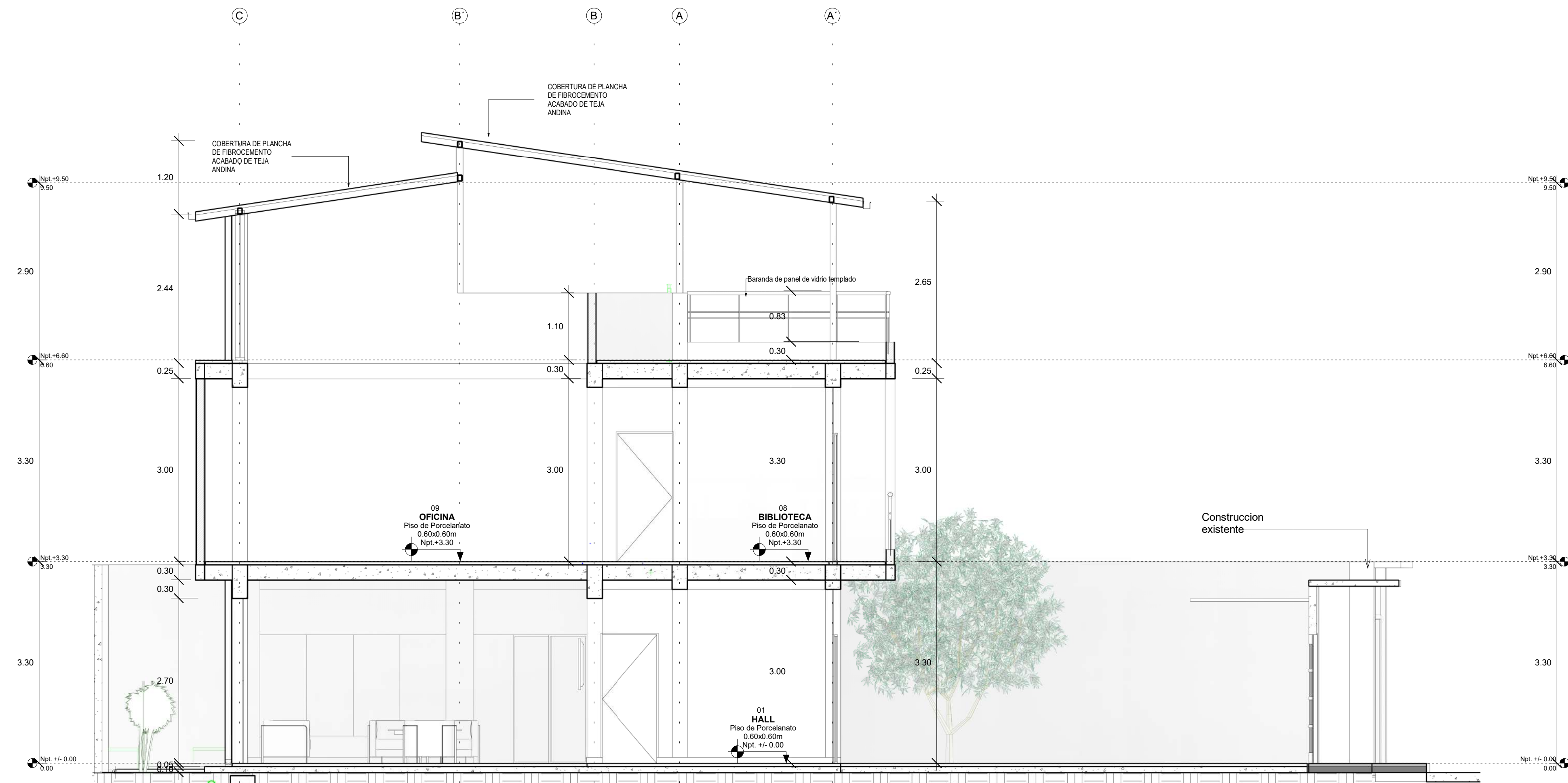
A CORTE LONGITUDINAL A-A A-04 1:50
