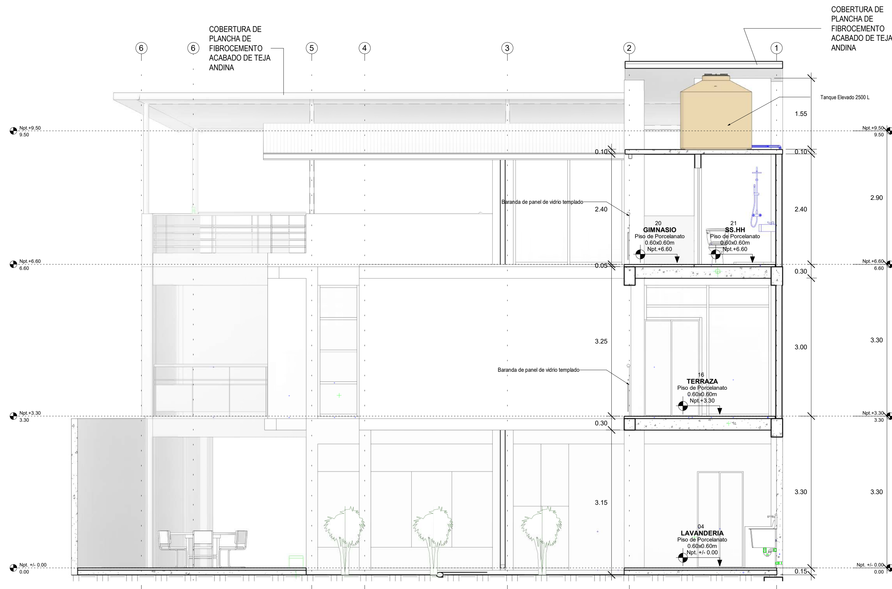
H CORTE TRANSVERSAL H-H A-06 1:50
