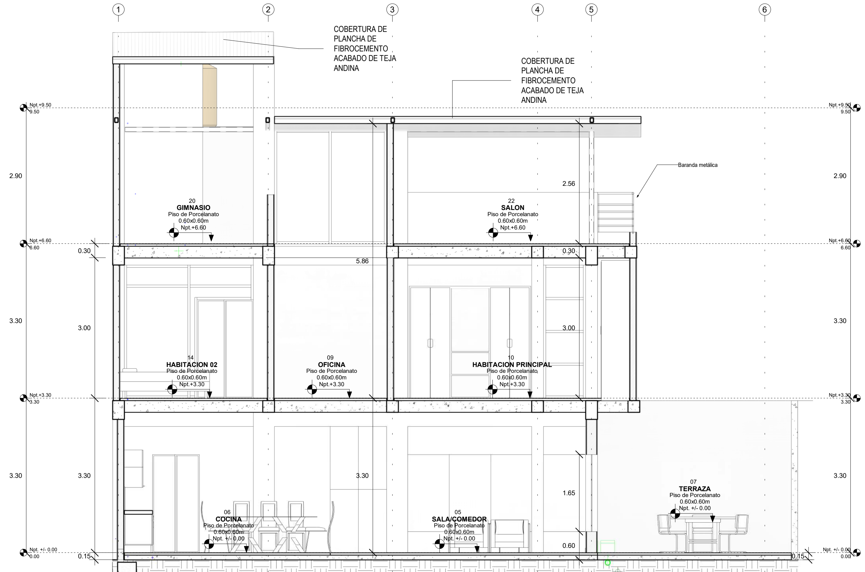
G CORTE TRANSVERSAL G-G A-06 1:50
