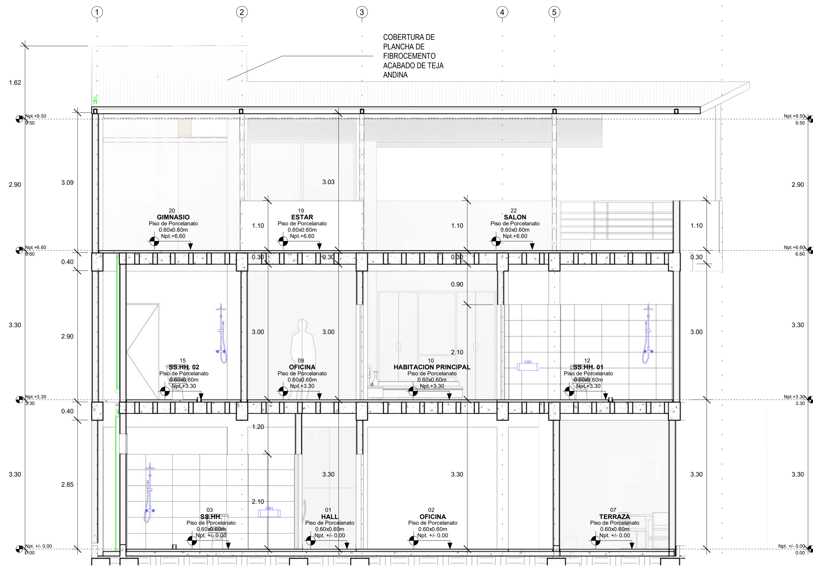
E CORTE TRANSVERSAL E-E A-05 1 : 50
