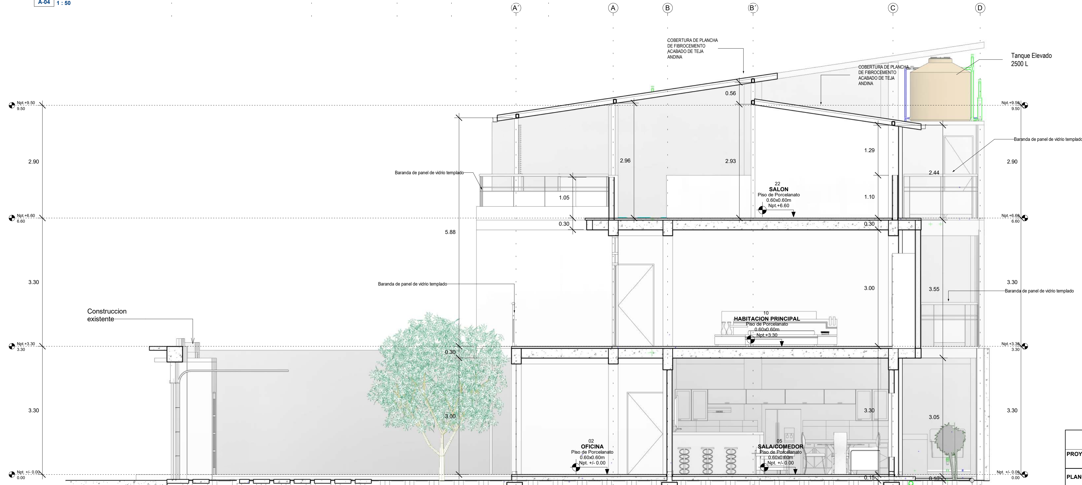
B CORTE LONGITUDINAL B-B A-04 1:50
