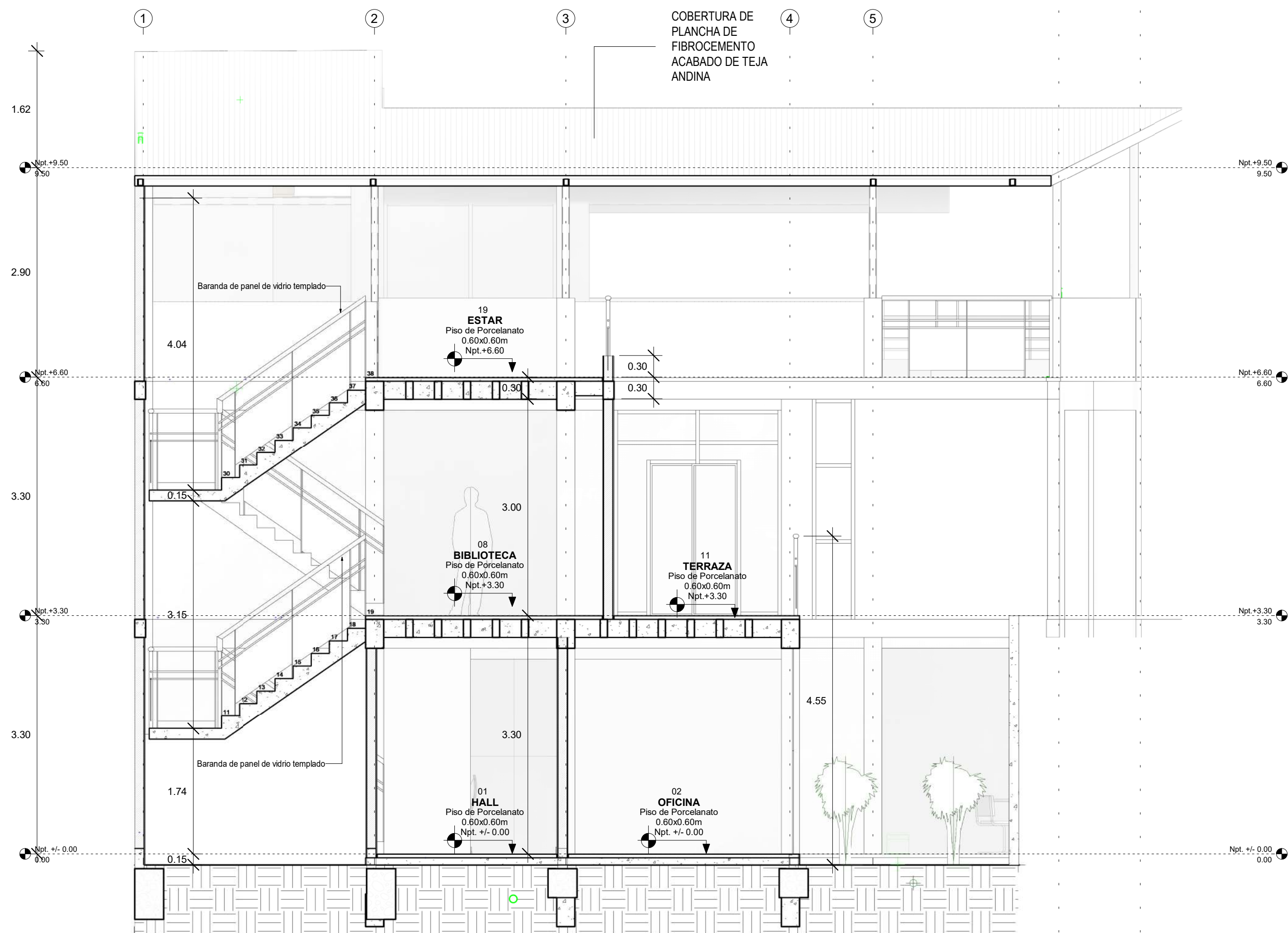
D CORTE TRANSVERSAL D-D A-05 1 : 50
