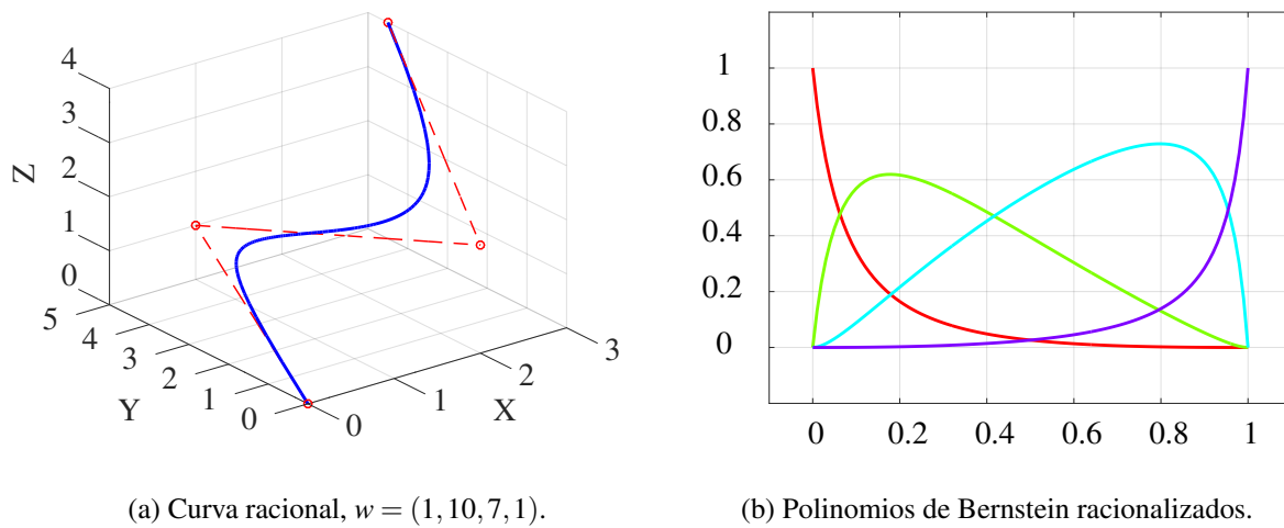
Figura 2.2: Curva de Bézier racionalizada junto a sus funciones base asociadas.
