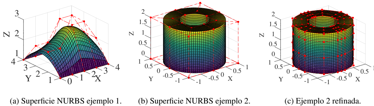
Figura 2.5: Ejemplos de distintas superficies NURBS
