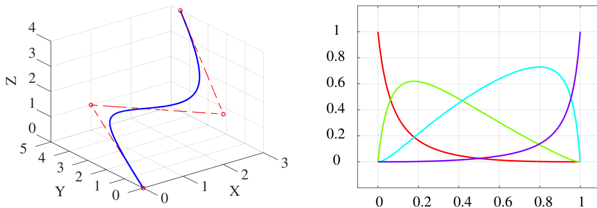
(a) Curva de Bézier de la figura 2.1a racionalizada con pesos w = (1, 10, 7, 1) . (b) Polinomios de Bernstein de la figura 2.1b racionalizados.
