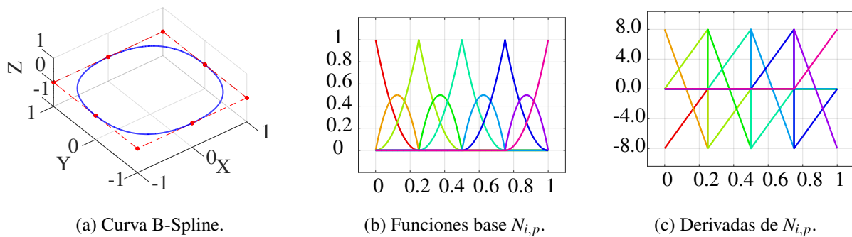
Figura 2.3: Curvas de Spline junto a sus funciones base y las derivadas de estas.
