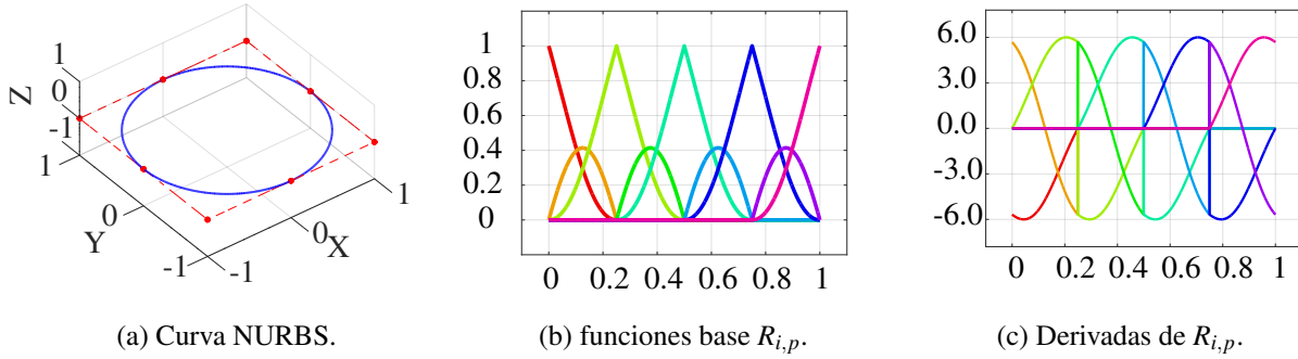
Figura 2.4: Curva NURBS con sus funciones base y las derivadas de estas.
