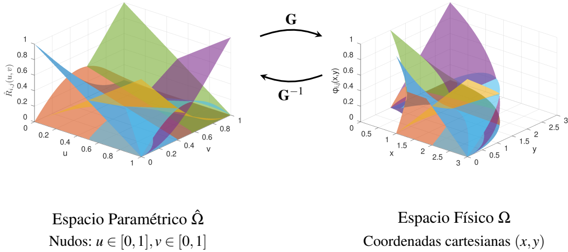
Figura 3.2: Correspondencia de las funciones de forma NURBS de la figura 3.1. Las funciones paramétricas \hat{R}_{i,j}^{p,q}(u, v) se definen inicialmente sobre el espacio para \hat{\Omega} (izquierda). Mediante el mapeo geométrico \mathbf{G} , el soporte se proyecta hacia el espacio físico \Omega (derecha), dando lugar a las funciones físicas \phi_{i,j}(x, y) = (\hat{R}_{i,j}^{p,q} \circ \mathbf{G}^{-1})(x, y) .
