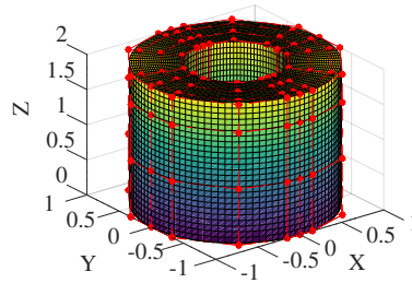
Figura 2.6: Superficie de la figura 2.5b tras inserción de nudos
