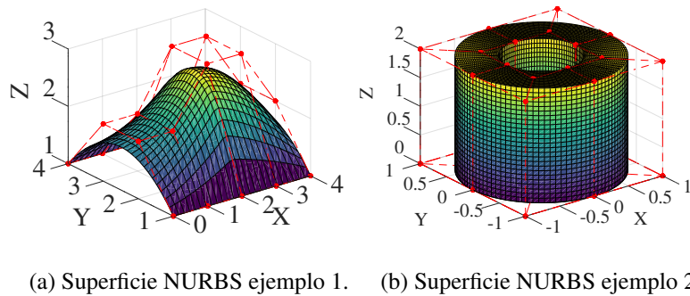
Figura 2.5: Ejemplos de distintas superficies NURBS
