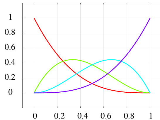
(b) Polinomios de Bernstein.
