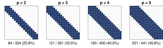
Figura 5.1: Elementos no nulos de la matriz frente al grado polinomial para N_{el} = 16 .
