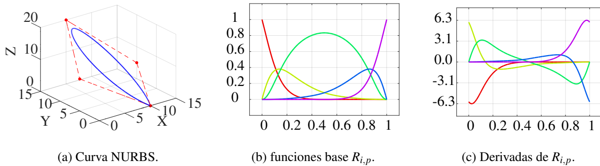
Figura 2.2: Curva NURBS con sus funciones base y las derivadas de estas.
