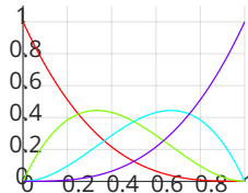
(c) Funciones base de Bernstein.
