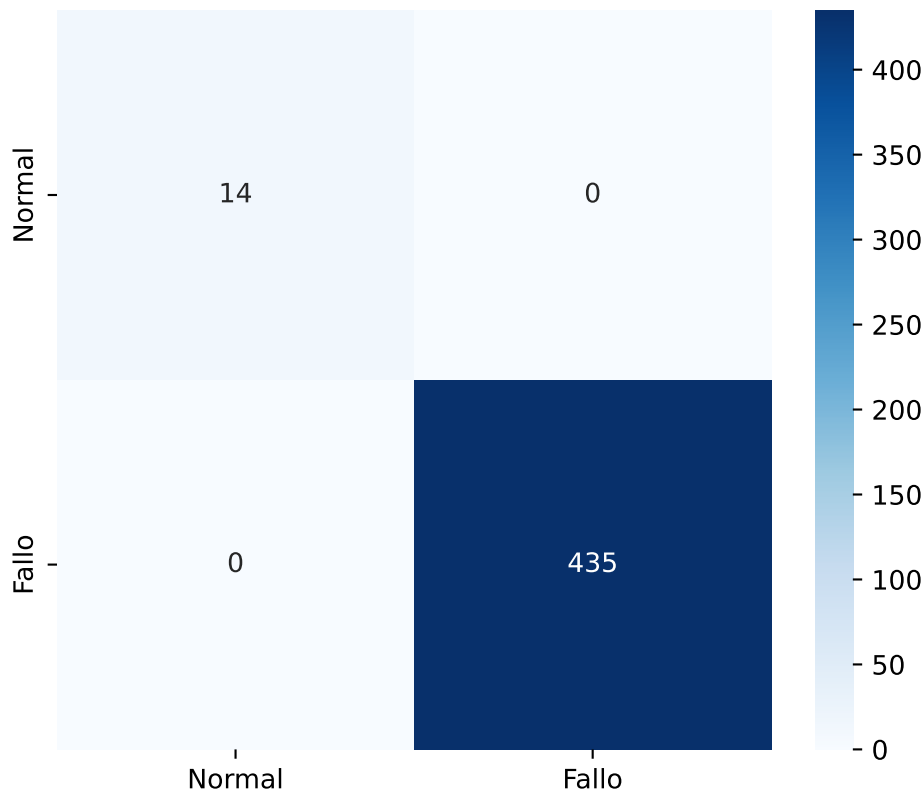
Matriz de Confusión MPE (Prueba)
