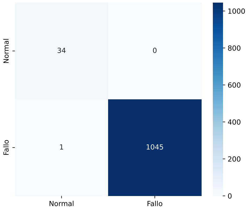
Matriz de Confusión MPE (Entrenamiento)
