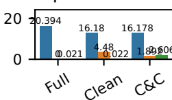
SpectralNorm
