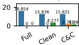
Microdown
