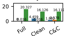
Fasta
