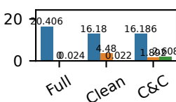
PiDigits
