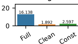
SpectralNorm
