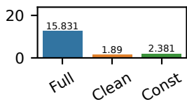
Microdown
