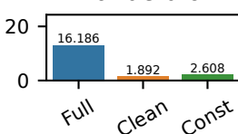
PiDigits
