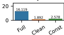
Fasta
