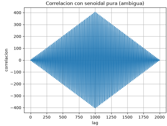
Fig. 3. Correlación cruzada utilizando una señal senoidal pura, mostrando ambigüedad periódica.
