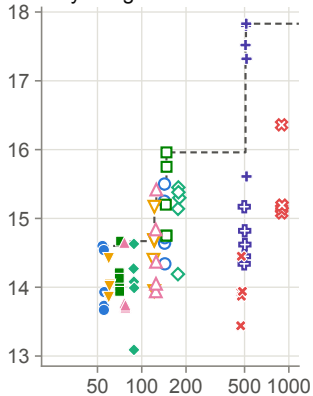
Tiny ImageNet
