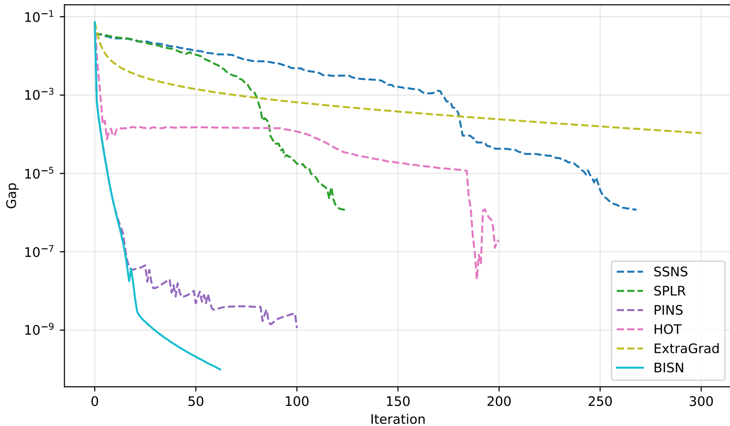
MNIST (ID1=0, ID2=1)
