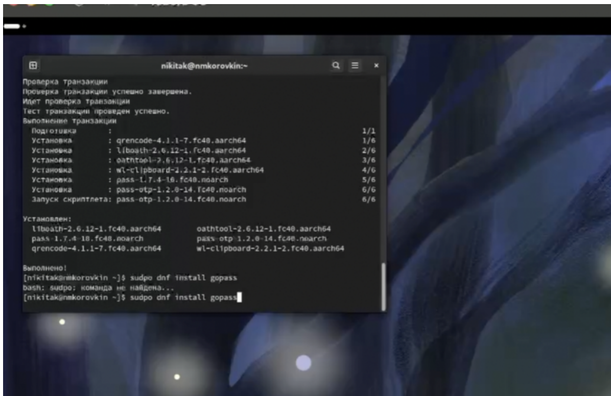
Рис. 3.2: Уставновим gopass
