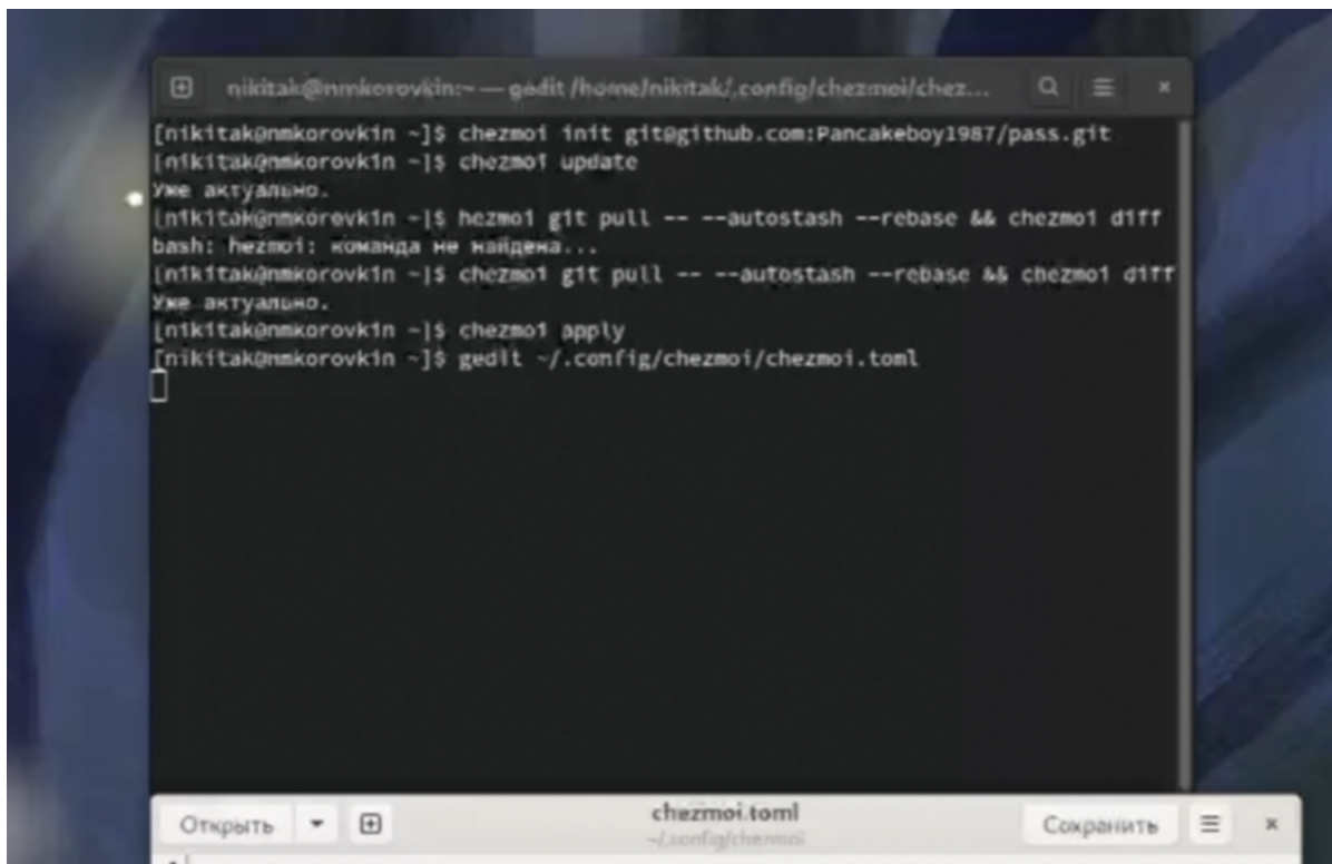
Рис. 3.8: настраиваем chezmoi
