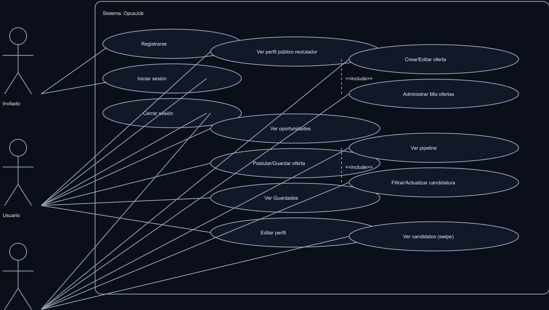
Diagrama UML de Casos de Uso — OpusJob
