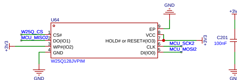
FLASH MEMORY W25Q128JVPIM
