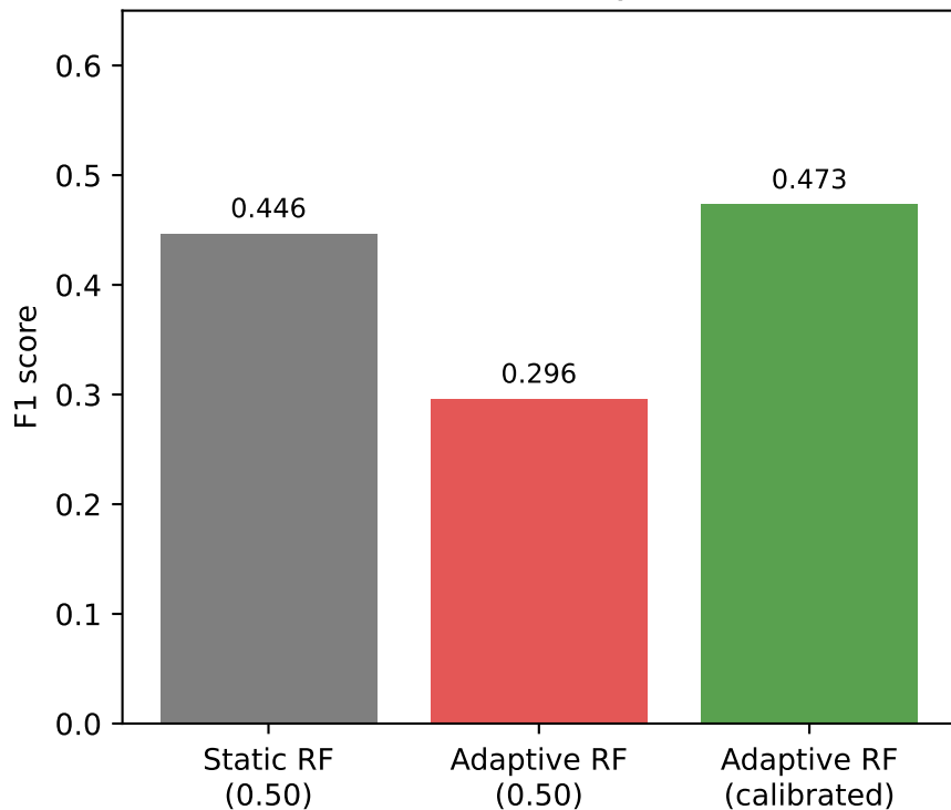
Held-out F1 (days 6-7)
