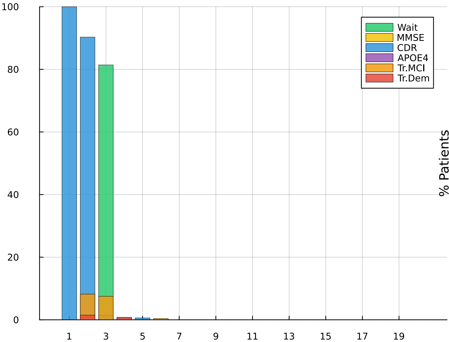
QMDP
