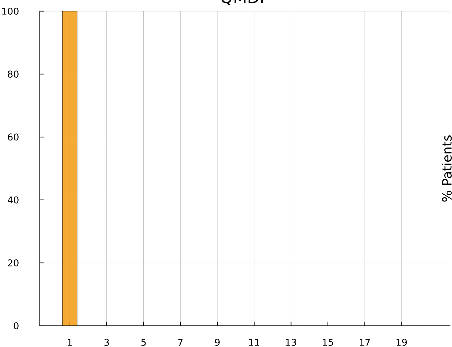
QMDP
