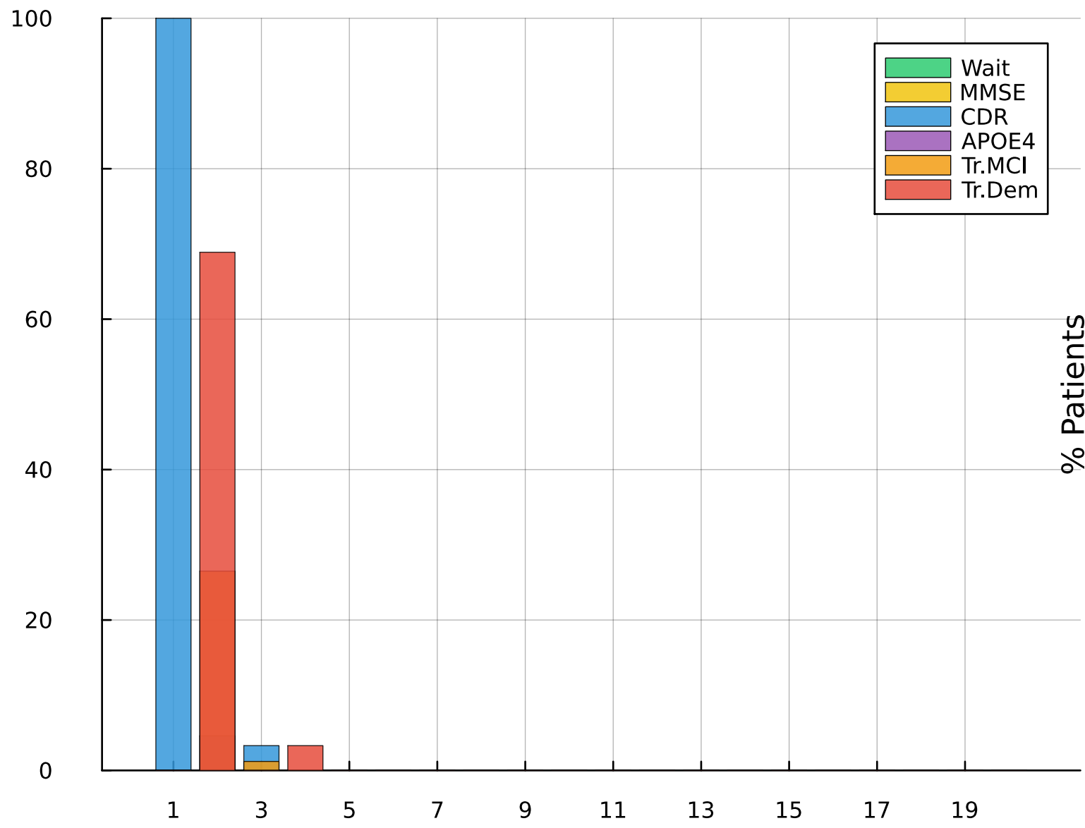
QMDP
